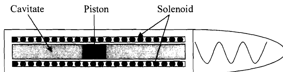
Secțiune longitudinală în dispozitivul (DN)
