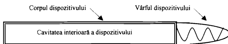
Fig. 3. Secțiune longitudinală în dispozitiv
