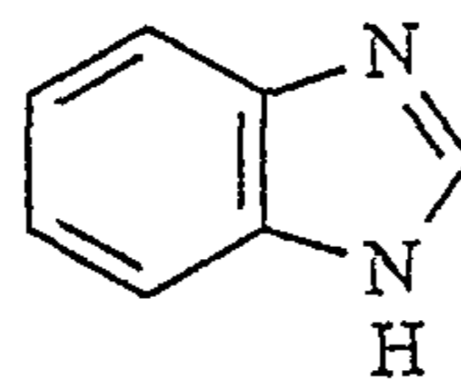
benzimidazole
