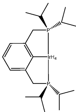
Complex 12: ( iPr PCP)IrH 4 ;
