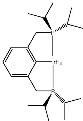
Complex 12: ( i\text{Pr}^4\text{PCP} )IrH 4 ;
