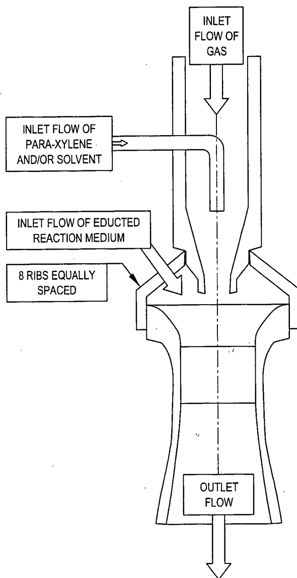
FIG. 27
