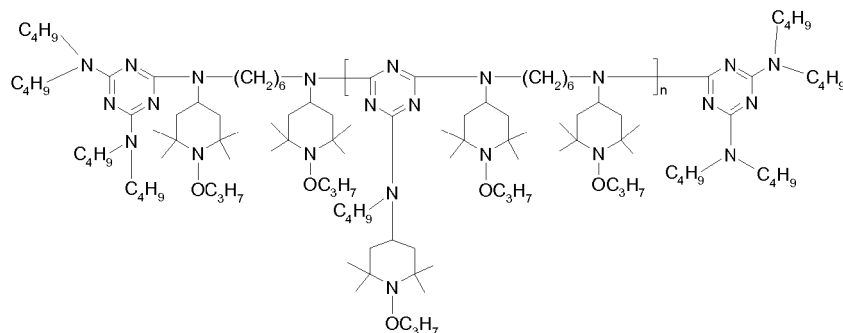
(Tinuvin®NOR 371)
