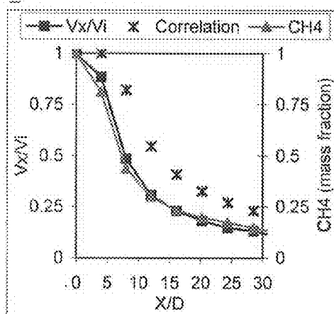
(d) d_{\text{air}}=0.3125 inch
