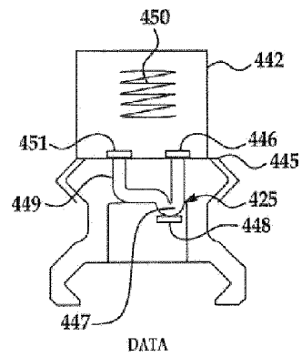
DATA FIG. 12A
