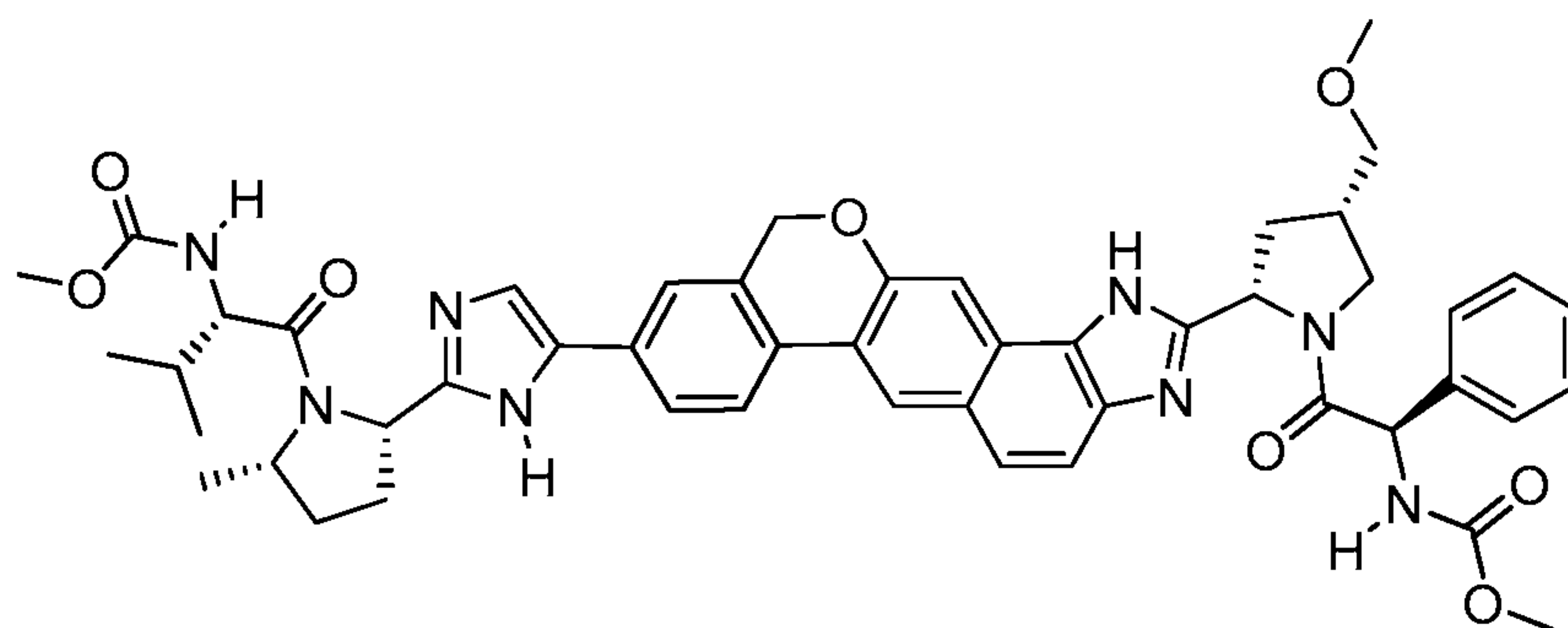
Methyl {(2S)-1-[(2S,5S)-2-(5-{2-[(2S,4S)-1-[(2R)-2-[(methoxycarbonyl)amino]-2-phenylacetyl]-4-(methoxymethyl)pyrrolidin-2-yl]-1,11 dihydroisochromeno [4',3':6,7]naphtho[1,2-d]imidazol-9-yl}-1H-imidazol-2-yl)-5-methylpyrrolidin-1-yl]-3-methyl-1-oxobutan-2-yl}carbamate
