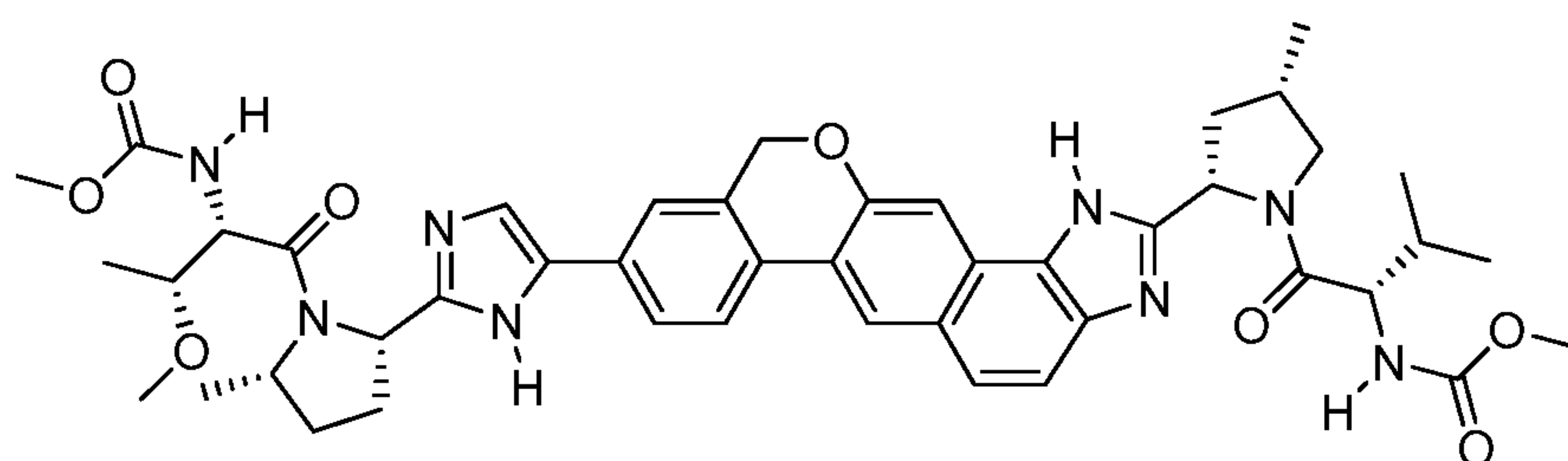
methyl [(2S)-1-{(2S,4S)-2-[9-(2-{(2S,5S)-1-[N-(methoxycarbonyl)-O-methyl-L-threonyl]-5-methylpyrrolidin-2-yl]-1H-imidazol-5-yl)-1,11-dihydroisochromeno[4',3':6,7]naphtho[1,2-d]imidazol-2-yl]-4-methylpyrrolidin-1-yl]-3-methyl-1-oxobutan-2-yl} carbamate
