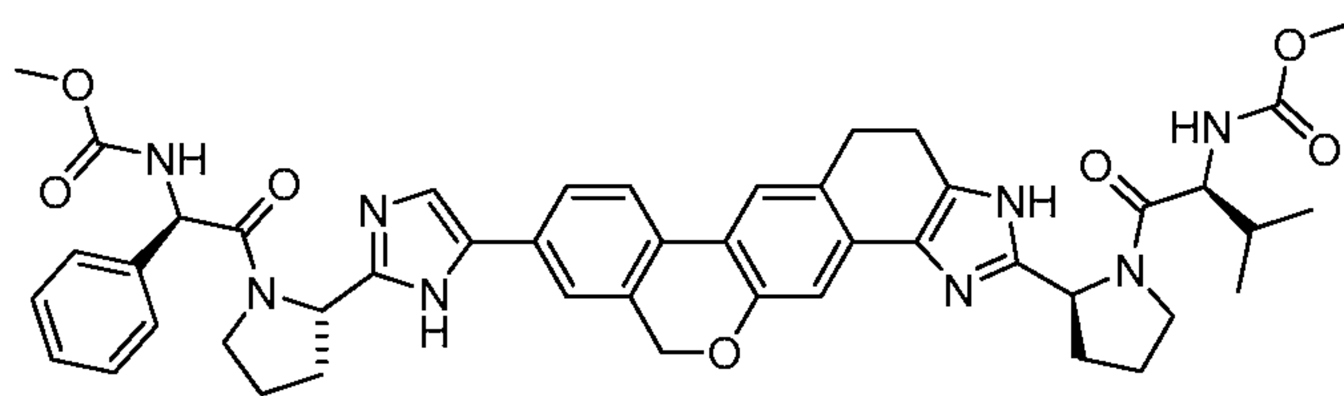
methyl [1-(2-{5-[2-(1-((methoxycarbonyl)amino)-3-methyl-1-oxobutan-2-yl})pyrrolidin-2-yl)-1,4,5,11-tetrahydroisochromeno[4',3':6,7]naphtho[1,2-d]imidazol-9-yl]-1H-imidazol-2-yl}pyrrolidin-1-yl)-phenyl-1-oxoacet-2-yl]carbamate
