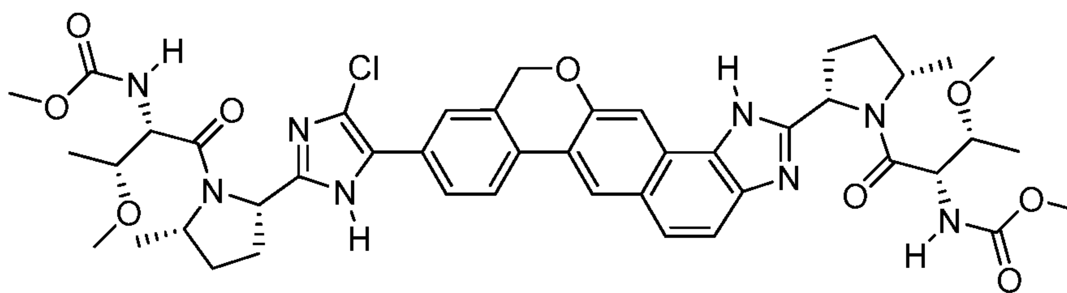
methyl [(2S,3R)-1-((2S,5S)-2-[9-(4-chloro-2-((2S,5S)-1-[N-(methoxycarbonyl)-O-methyl-L-threonyl]-5-methylpyrrolidin-2-yl)-1H-imidazol-5-yl)-1,11-dihydroisochromeno[4',3':6,7]naphtho[1,2-d]imidazol-2-yl]-5-methylpyrrolidin-1-yl]-3-methoxy-1-oxobutan-2-yl]carbamate
