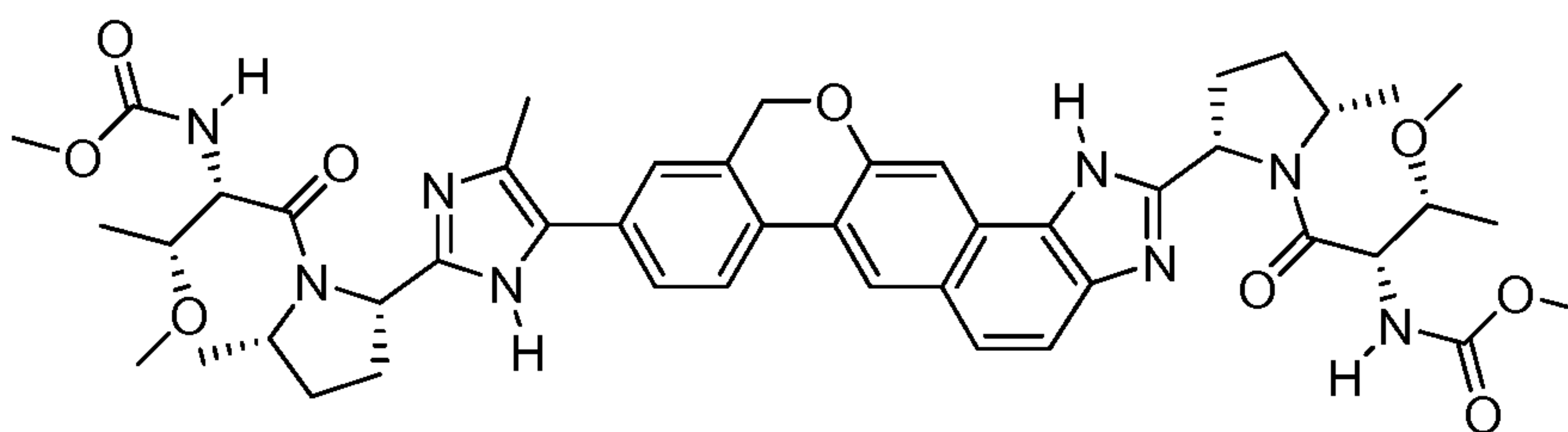
methyl [(2S,3R)-3-methoxy-1-{(2S,5S)-2-[9-(2-{(2S,5S)-1-[N-(methoxycarbonyl)-O-methyl-L-threonyl]-5-methylpyrrolidin-2-yl]-4-methyl-1H-imidazol-5-yl)-1,11-dihydroisochromeno[4',3':6,7]naphtho[1,2-d]imidazol-2-yl]-5-methylpyrrolidin-1-yl}-1-oxobutan-2-yl]carbamate
