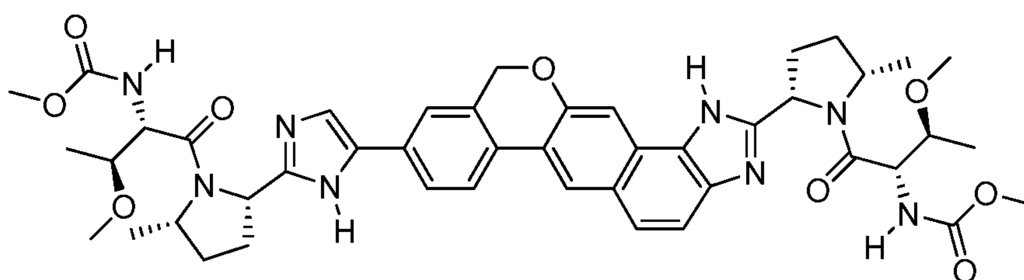
methyl [(2S,3S)-3-methoxy-1-{(2S,5S)-2-[9-(2-{(2S,5S)-1-[N-(methoxycarbonyl)-O-methyl-L-allothreonyl]-5-methylpyrrolidin-2-yl]-1H-imidazol-5-yl)-1,11-dihydroisochromeno[4',3':6,7]naphtho[1,2-d]imidazol-2-yl]-5-methylpyrrolidin-1-yl}-1-oxobutan-2-yl]carbamate
