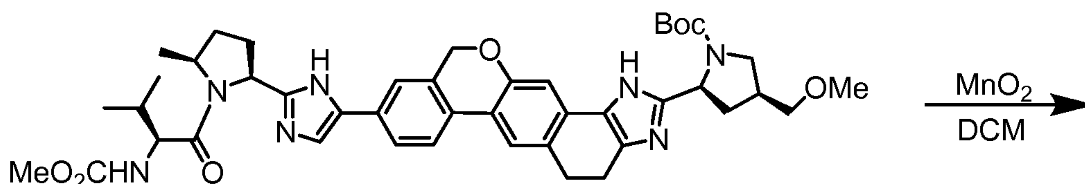
tert-butyl (2S,4S)-2-[9-(2-{(2S,5S)-1-[N-(methoxycarbonyl)-L-valyl]-5-methylpyrrolidin-2-yl}-1H-imidazol-5-yl)-1,4,5,11-tetrahydroisochromeno[4',3':6,7]naphtho[1,2-d]imidazol-2-yl]-4-(methoxymethyl)pyrrolidine-1-carboxylate
