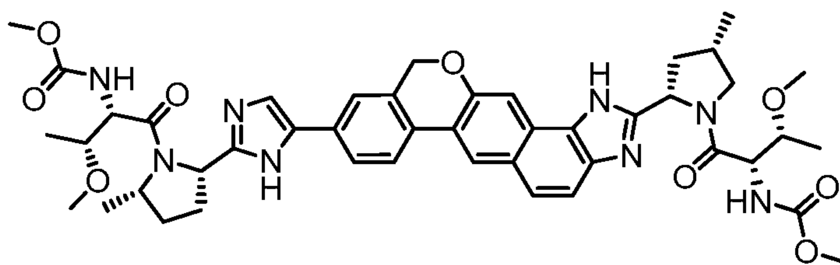
methyl [(2S,3R)-3-methoxy-1-{(2S,5S)-2-[9-(2-{(2S,5S)-1-[N-(methoxycarbonyl)-O-methyl-L-threonyl]-5-methylpyrrolidin-2-yl]-1H-imidazol-5-yl)-1,11-dihydroisochromeno[4',3':6,7]naphtho[1,2-d]imidazol-2-yl]-4-methylpyrrolidin-1-yl}-1-oxobutan-2-yl]carbamate
