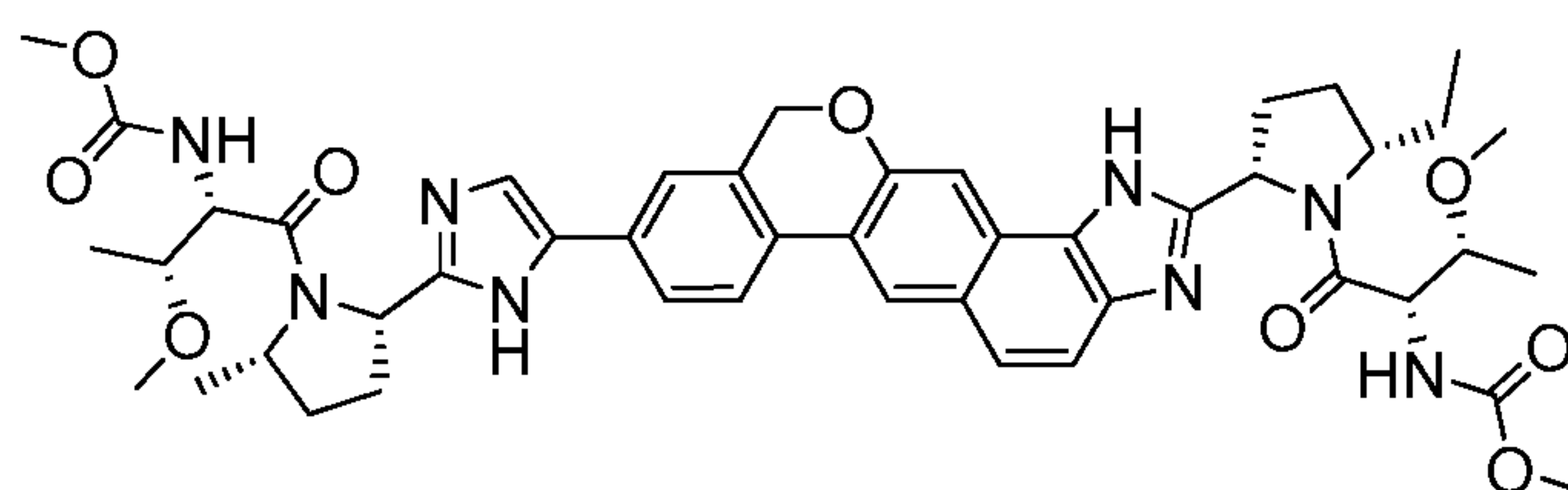
methyl[(2S,3R)-1-{(2S,5S)-2-[5-(2-{(2S,5S)-5-ethyl-1-[N-(methoxycarbonyl)-O-methyl-L-threonyl]pyrrolidin-2-yl})-1,11-dihydroisochromeno[4',3':6,7]naphtho[1,2-d]imidazol-9-yl)-1H-imidazol-2-yl]-5-methylpyrrolidin-1-yl}-3-methoxy-1-oxobutan-2-yl]carbamate
