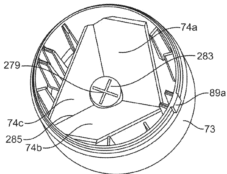
FIG. 7G
