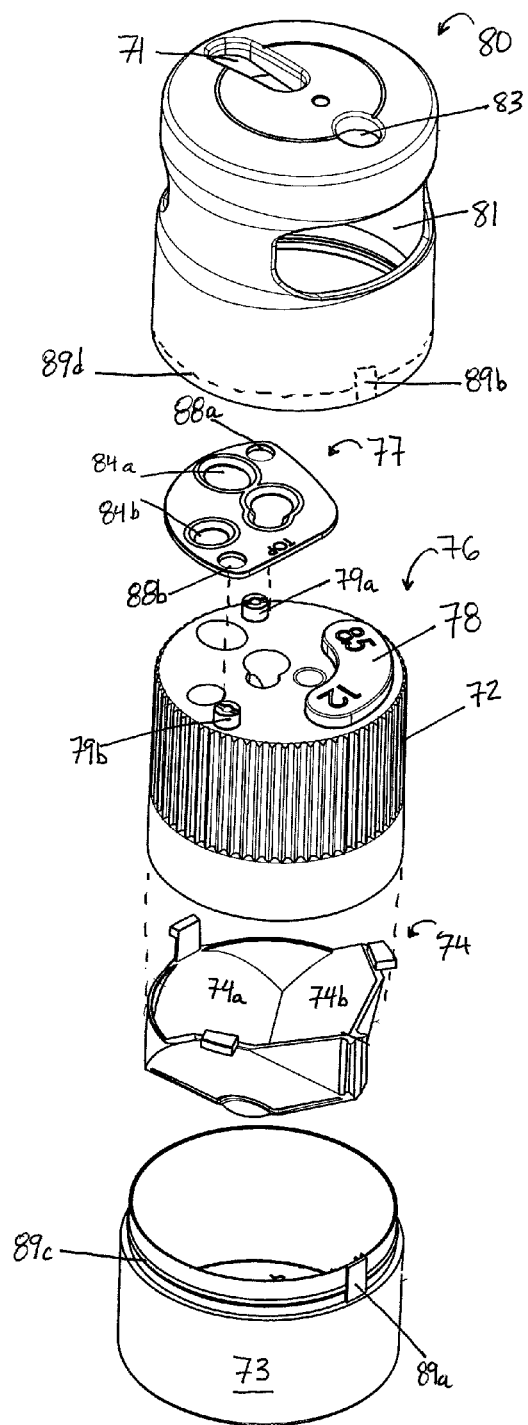
FIG. 3B
