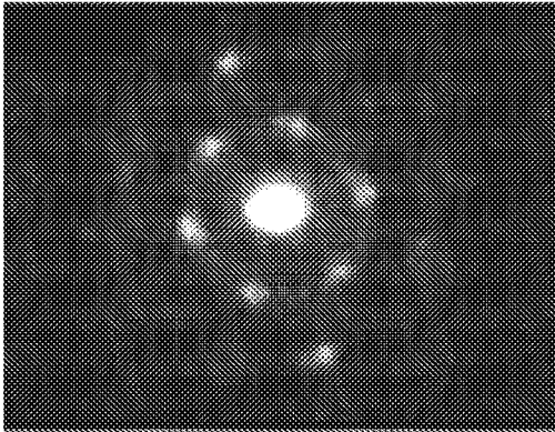
CAAC-OS
