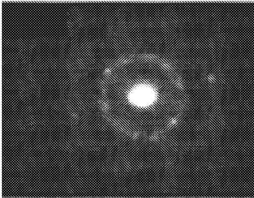
nc-OS
