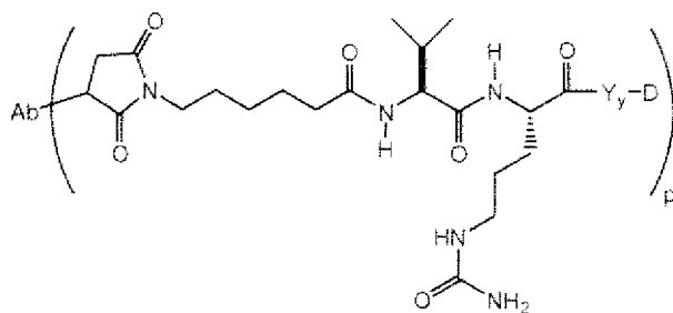
MC-val-cit
