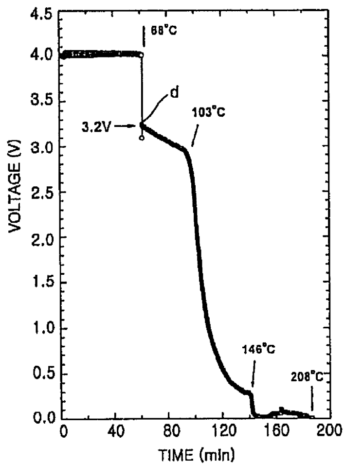
FIG. 5B
