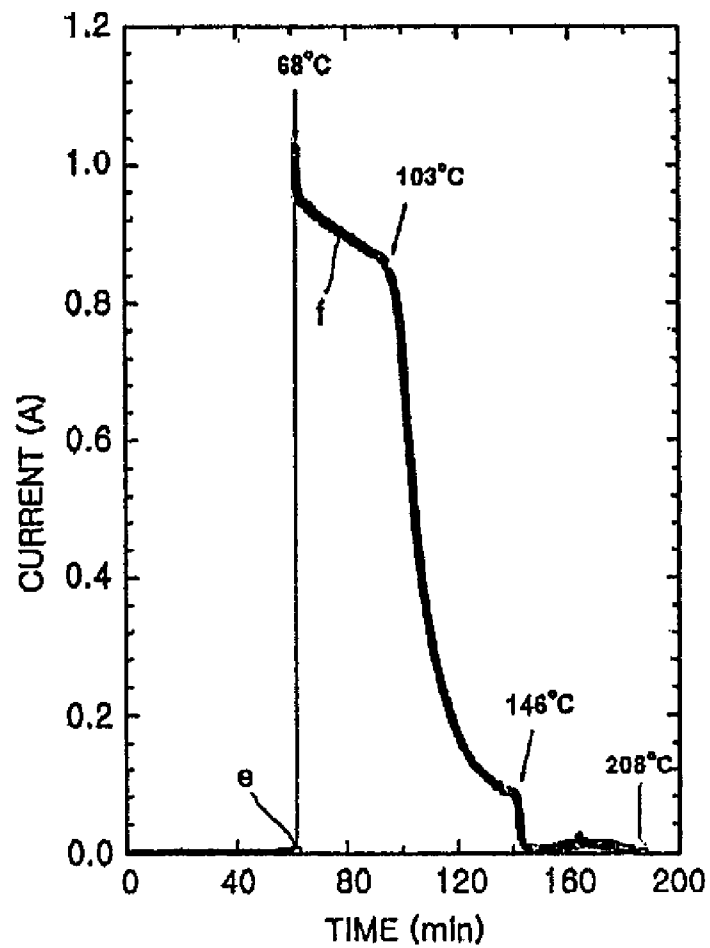
FIG. 5C
