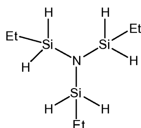
Tri(ethylsilyl)amine
