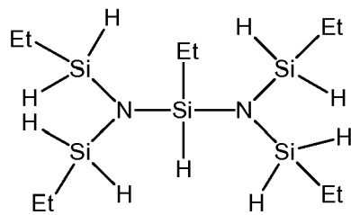
Bis(bis(ethylsilyl)amino)ethylsilane
