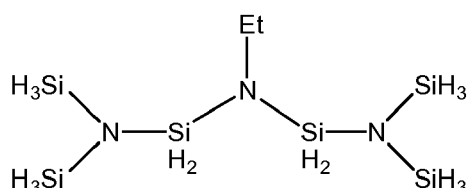
Bis[bis(ethylsilyl)amino)silyl]ethanamine
