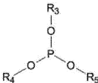
[Chemische Formel 2]
