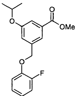
Compound (d)
