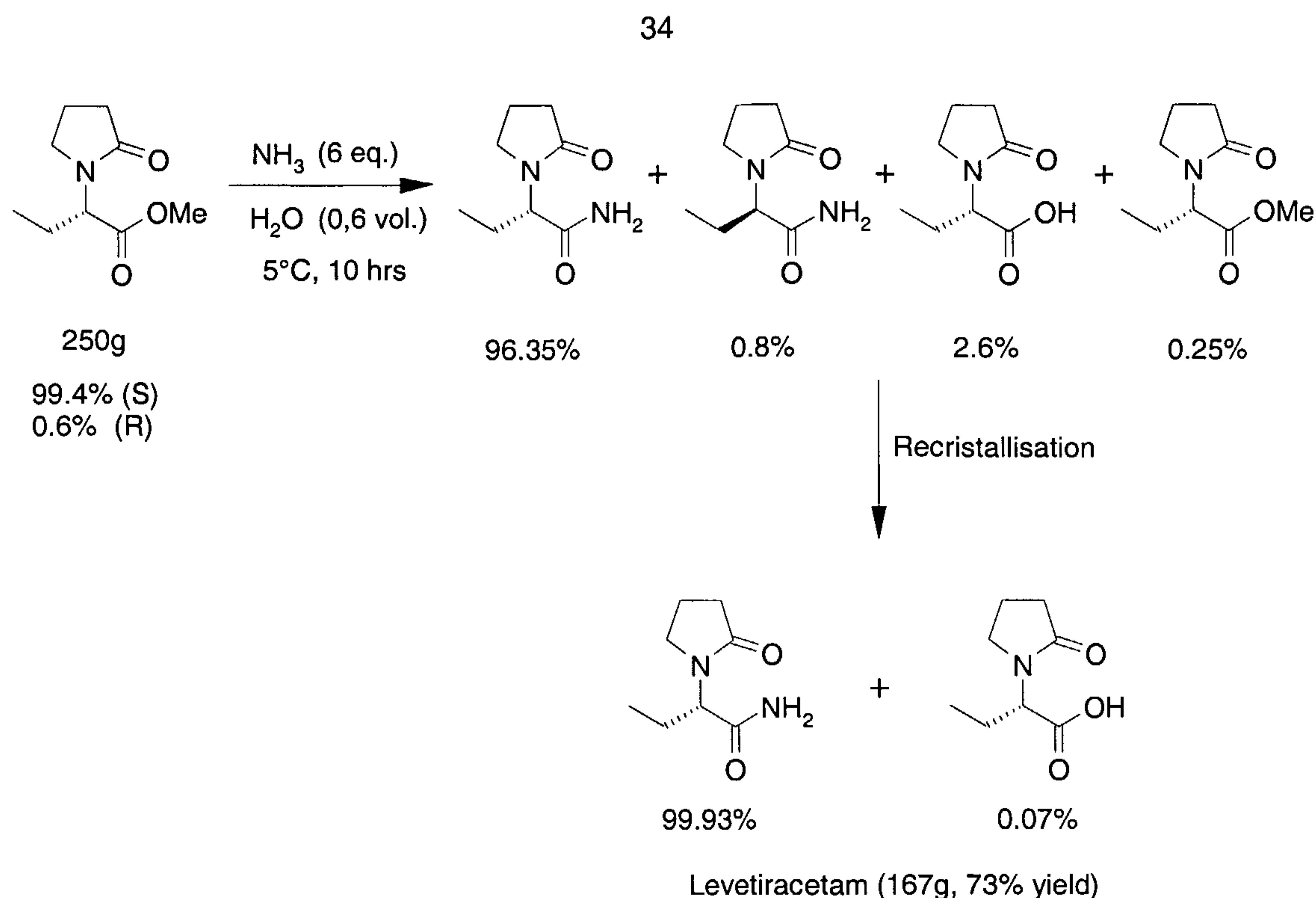
Scheme 18.
