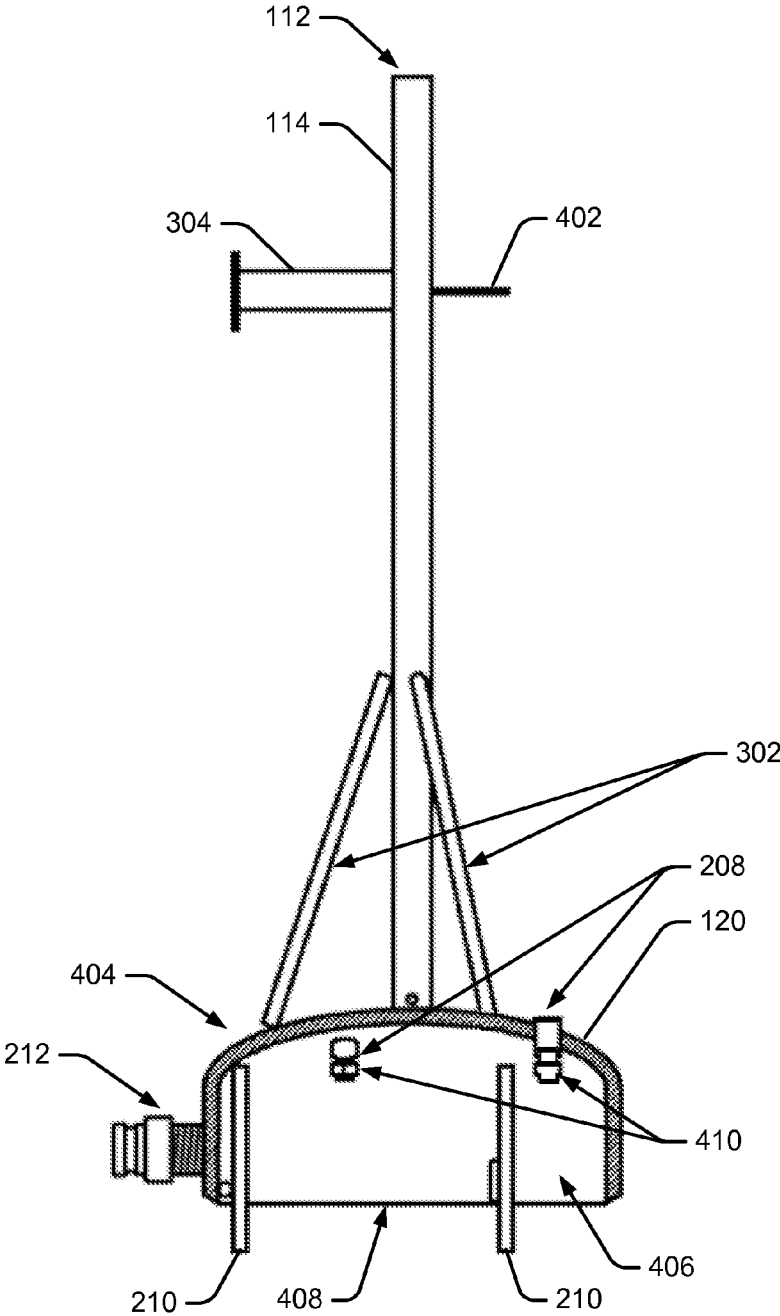
SECTION A-A
