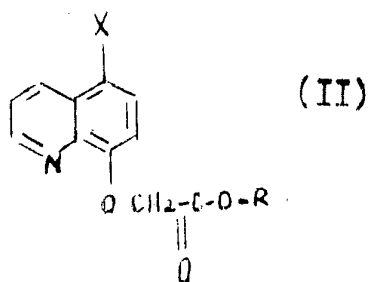
2-oji lentelė: Junginiai pagal II-ąją formulę
