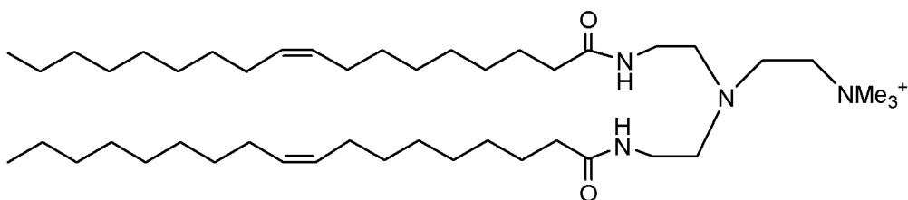
甲基-二油酰基单胺(6.1)
