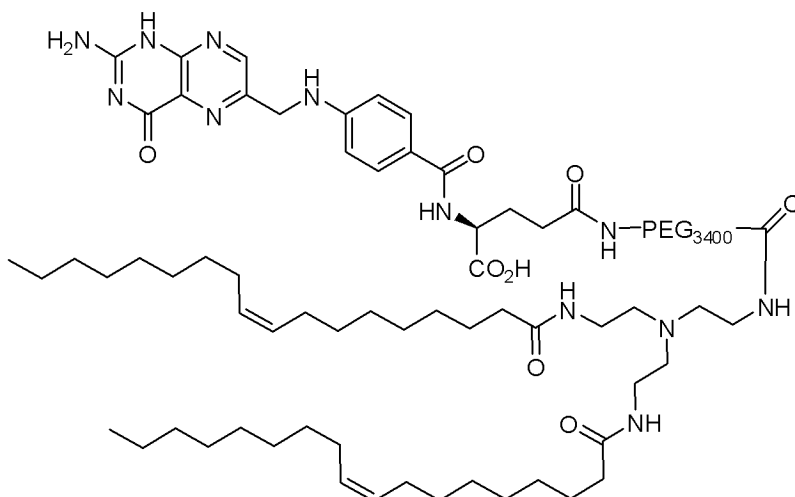
叶酸盐-PEG-二油酰基单胺(8)
