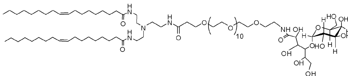
乳糖酰基-二油酰基单胺(10)
