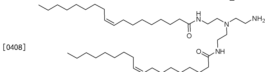
二油酰基单胺(6)
