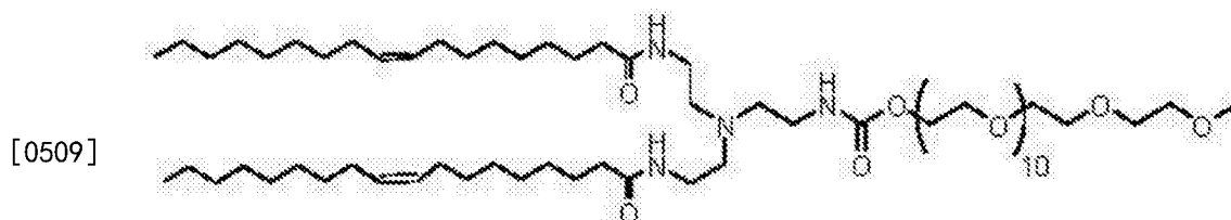
mPEG-二油酰基单胺(9)
