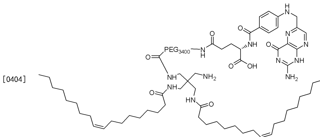
叶酸盐-PEG-二油酰基交叉胺(5)
