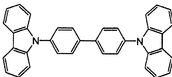
[Chem. 3]
