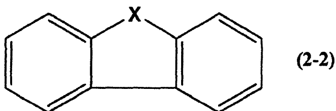
[Chem. 3]
