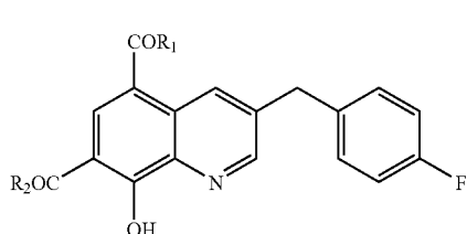
I-192~I-243
