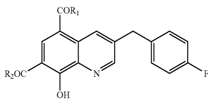
I-245~I-249
