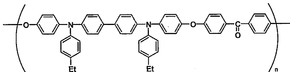
Et-PTPDEK
