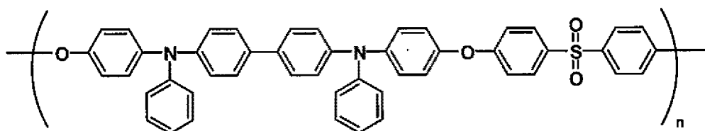
PTPDES
