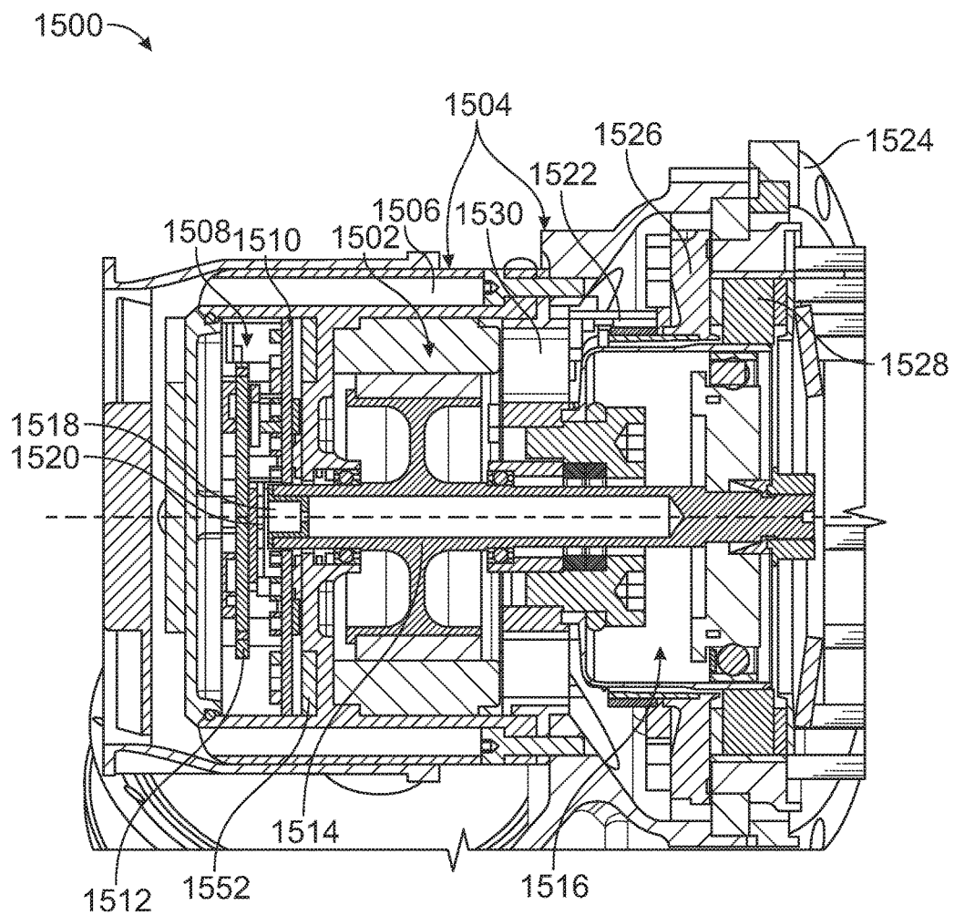
FIG. 15A
