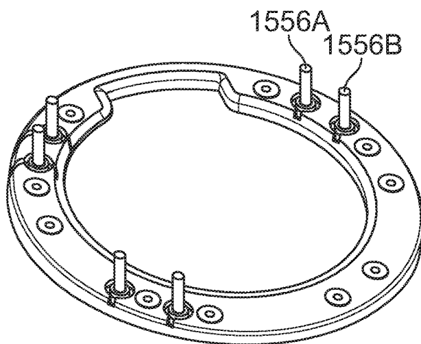
FIG. 15F
