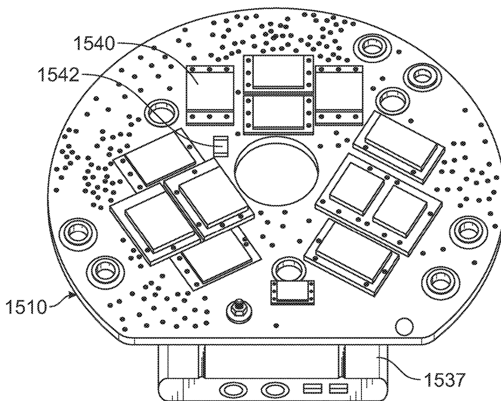
FIG. 15D
