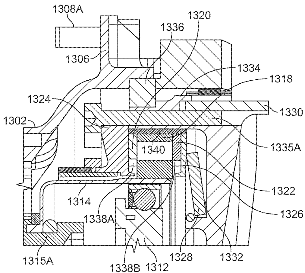
FIG. 13B
