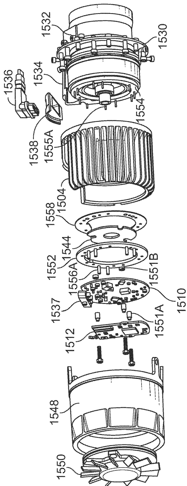
FIG. 15G
