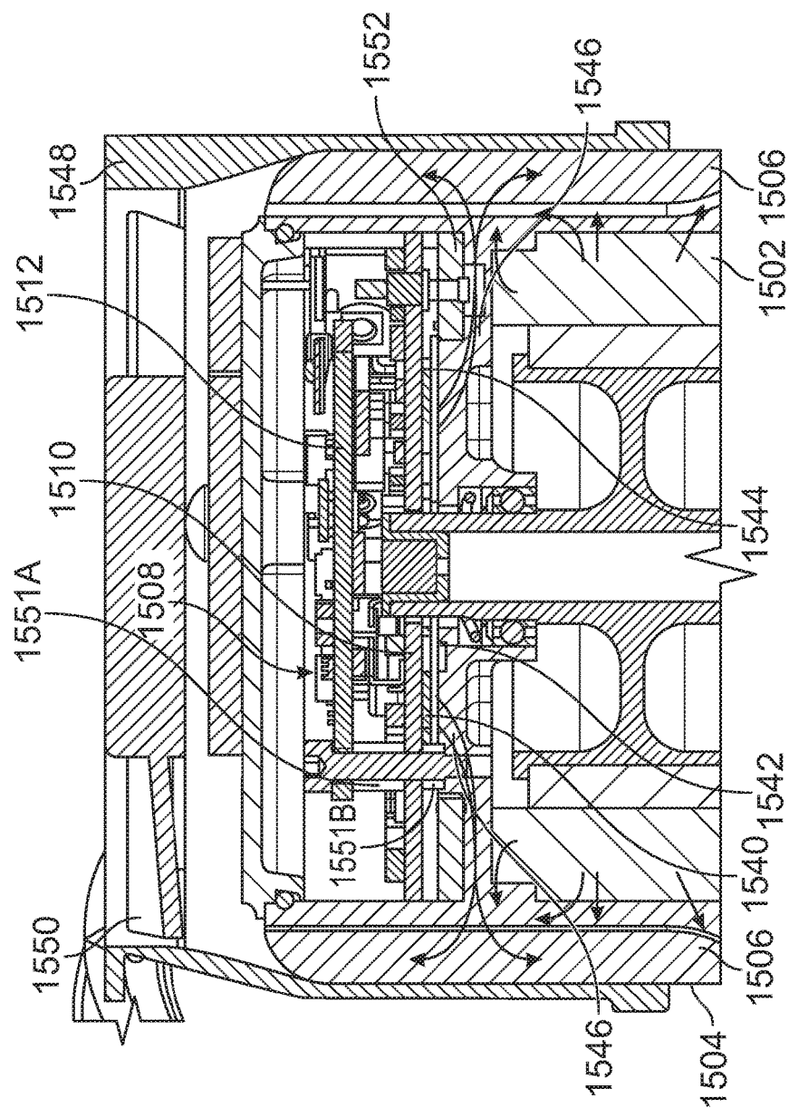
FIG. 15C
