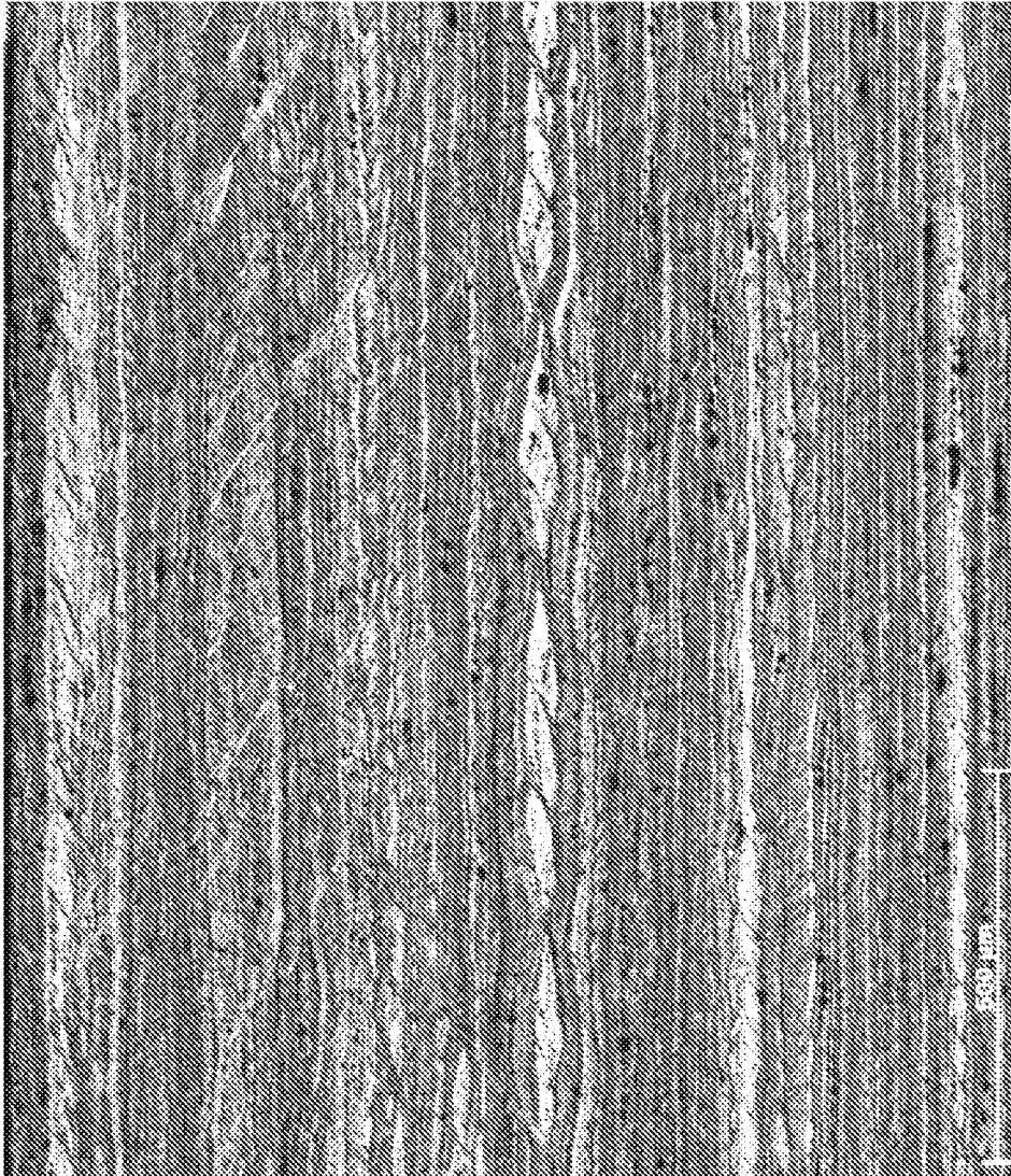
6xxx+Cu+Zn Aluminum Alloy – 85% CW FIG. 11e
