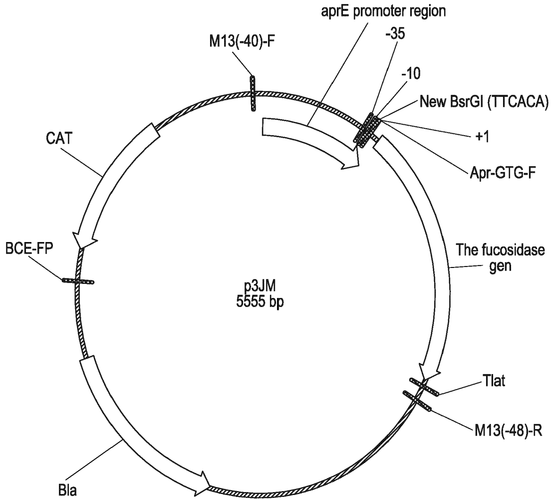
Exemplary plasmid map p3JM
