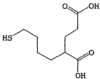
2-(4-sulfanylbutyl)pentanedioic acid
