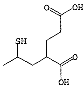
2-(2-sulfanylpropyl)pentanedioic acid
