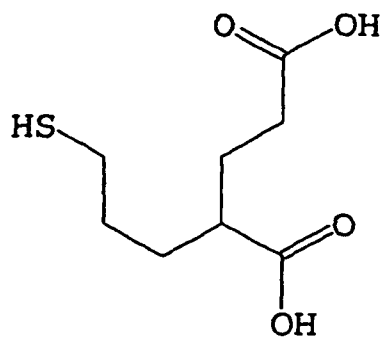
2-(3-sulfanylpropyl)pentanedioic acid
