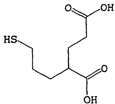
2-(3-sulfanylpropyl)pentanedioic acid
