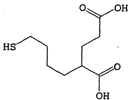
2-(4-sulfanylbutyl)pentanedioic acid
