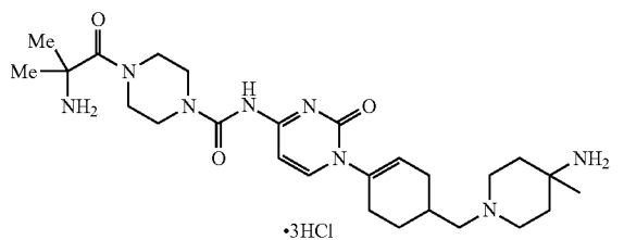
Enantiomer 2
