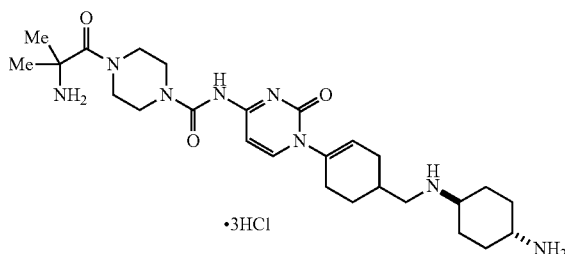
Enantiomer 2
