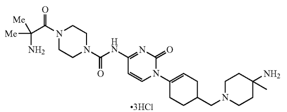
Enantiomer 2
