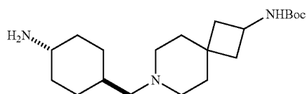
tert-Butyl (7-((trans-4-aminocyclohexyl)methyl)-7-azaspiro[3.5]nonan-2-yl)carbamate
