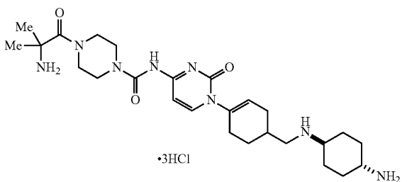
Enantiomer 1
