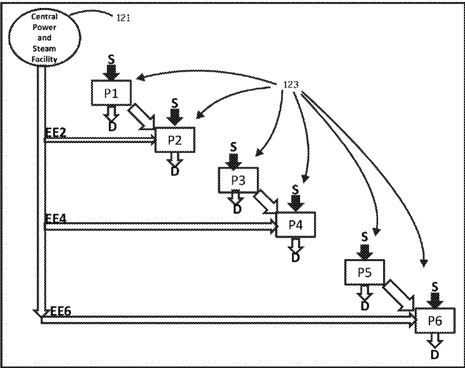
FIG. 21. (PRIOR ART)
