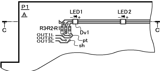
[B]第2面(裏面)側のパターン図
