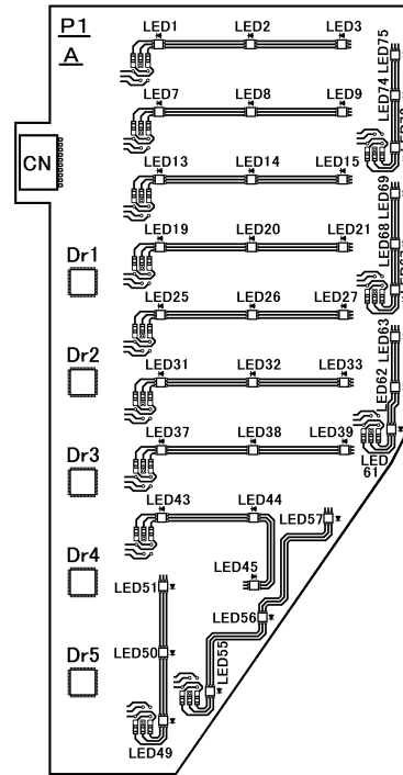
[A]第1面(表面)側
