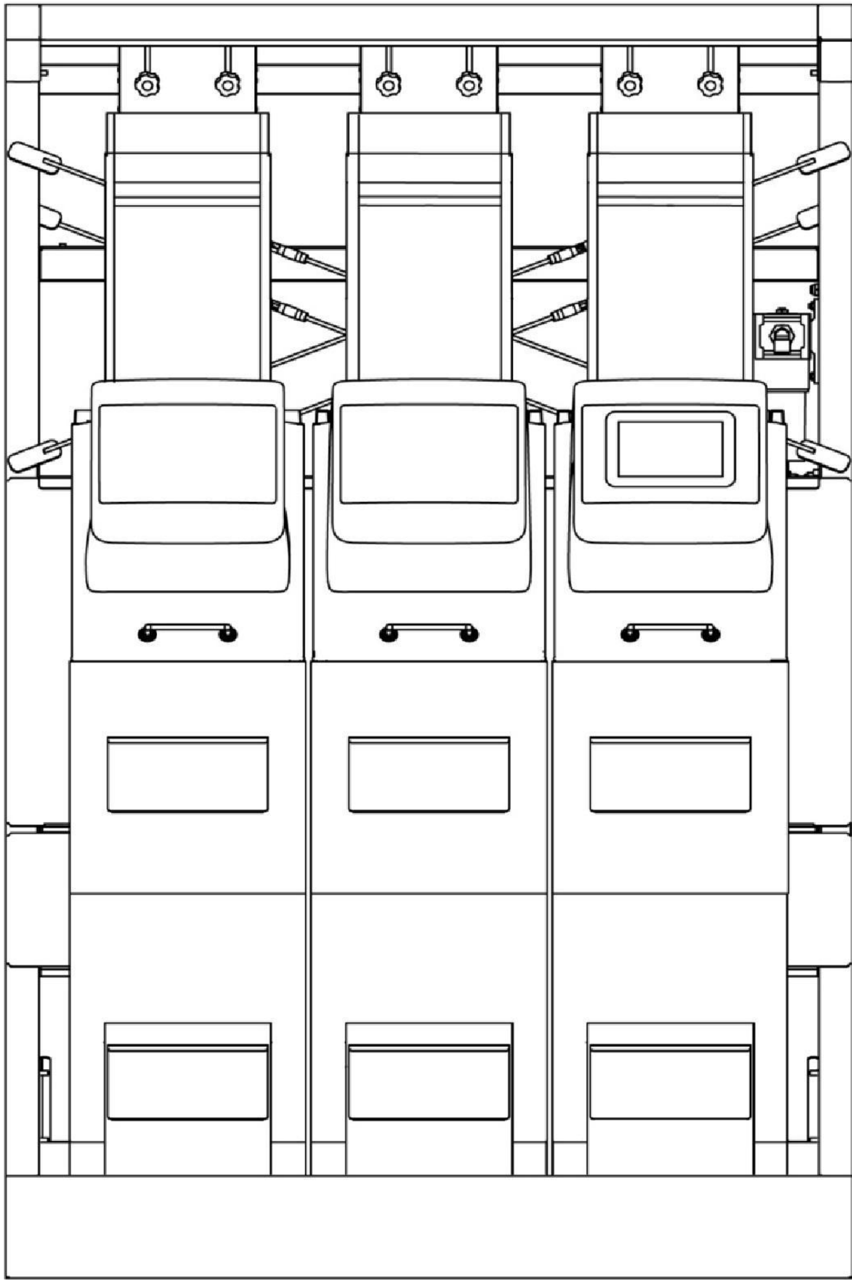
【前視圖】
