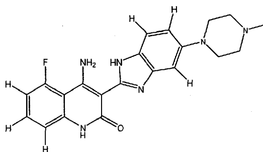
Tautomer IIIBb
