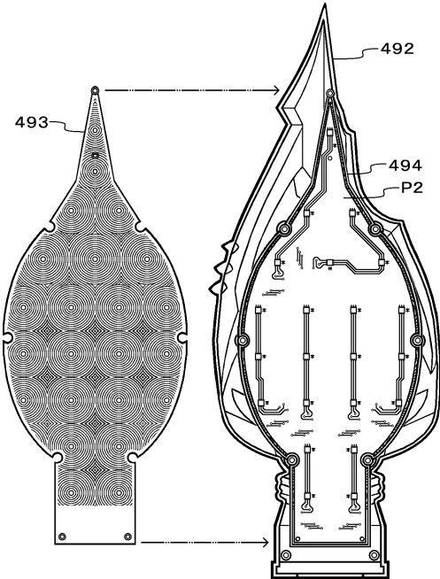
組立図2 fig.240
