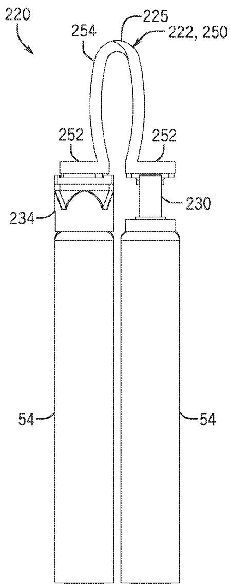
FIG. 35
