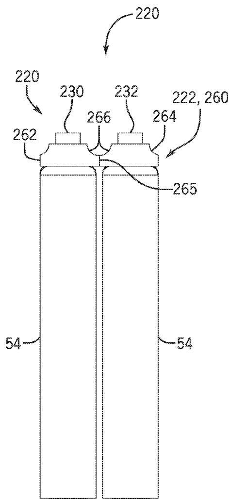
FIG. 36
