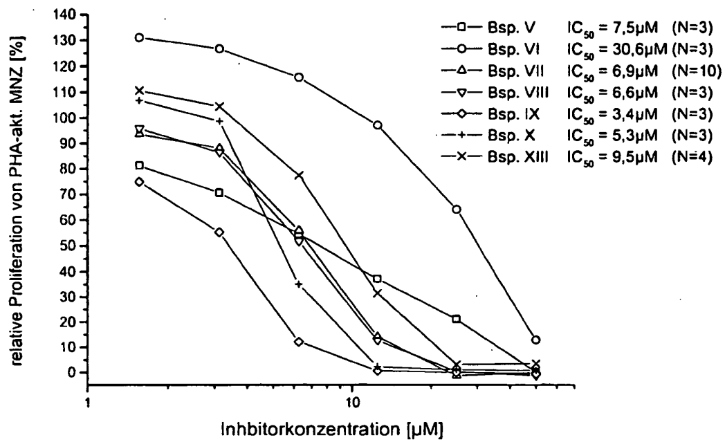
Figur 1: Hemmung der Phytohämagglutinin-induzierten Proliferation mononukleärer Zellen (MNZ) gesunder Spender durch in Tabelle 3 und 4 aufgeführte Substanzbeispiele (V – XIII).
