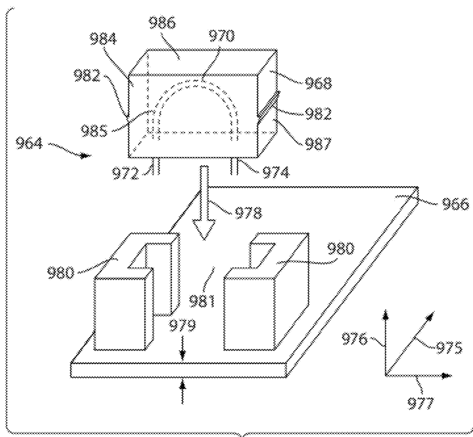
Fig. 14A
