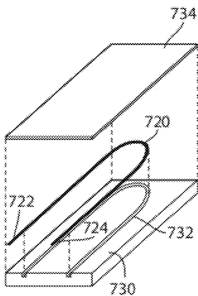
Fig. 8C
