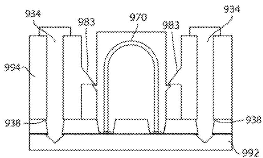
Fig. 16B
