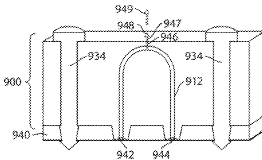
Fig. 12E
