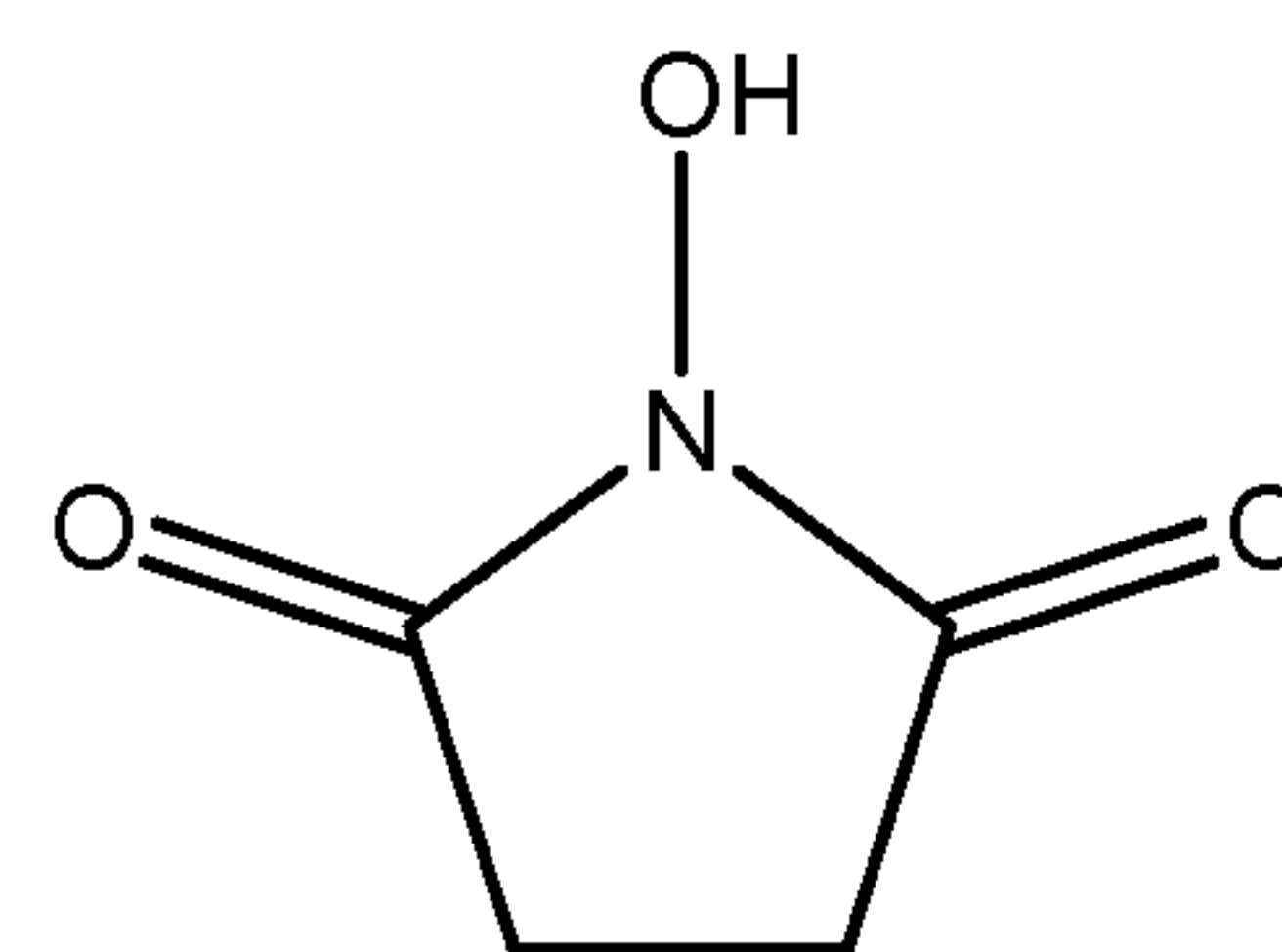
NHS
