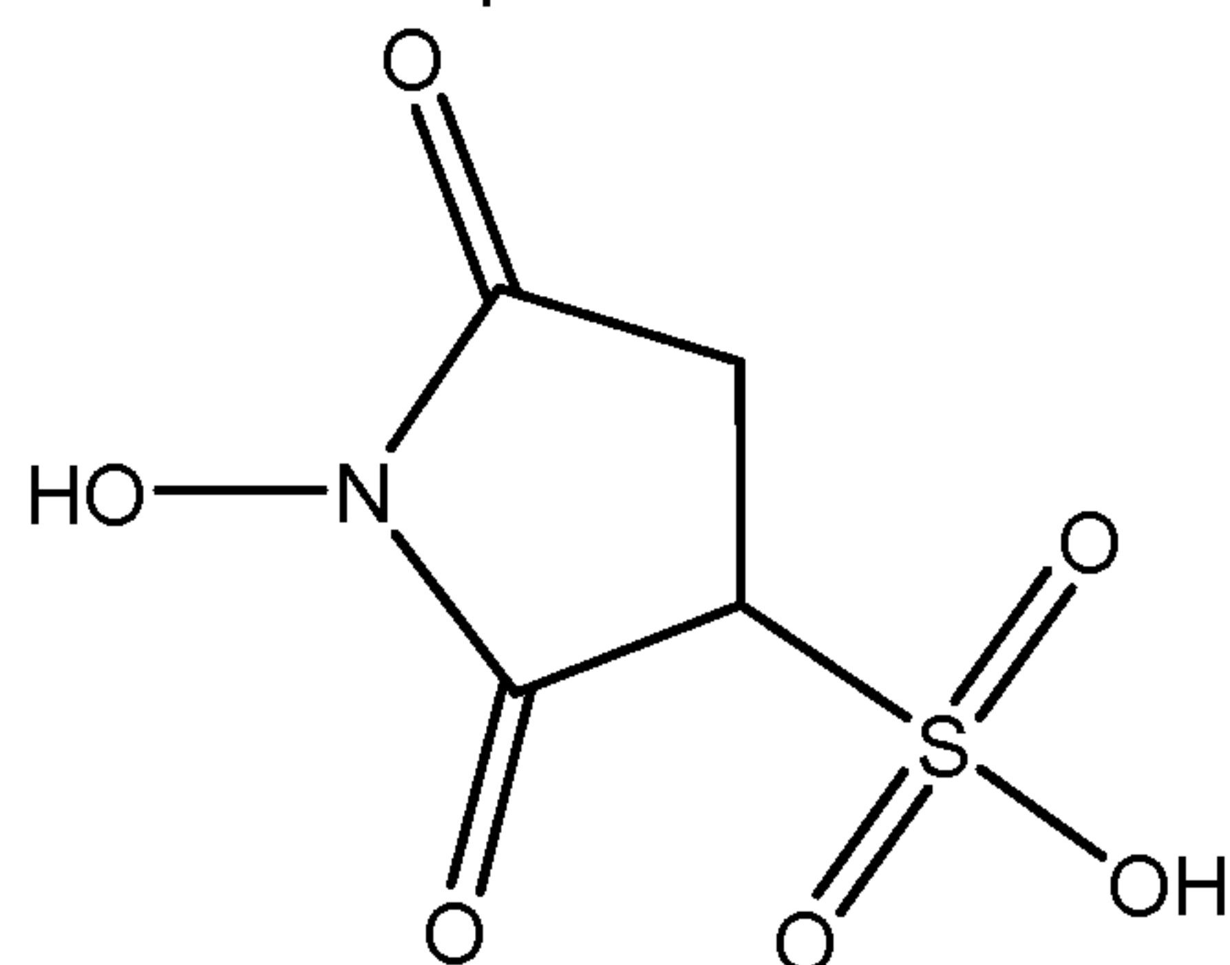
sulfoNHS
