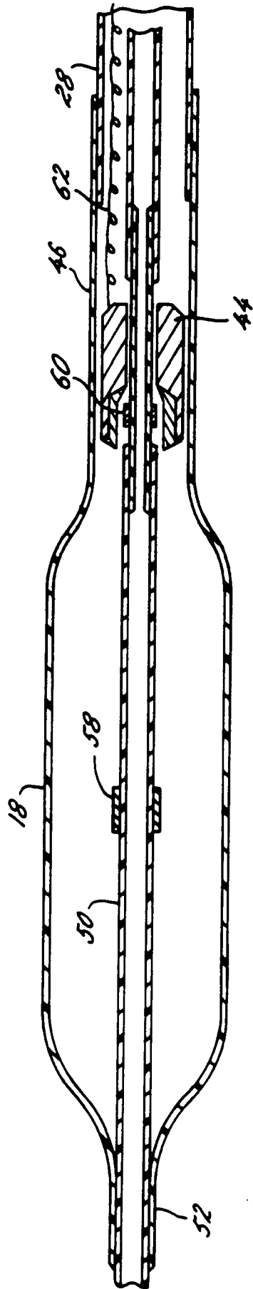
FIG. 3a
