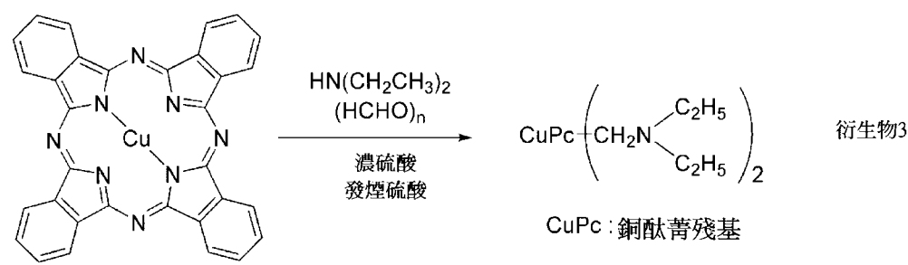
[化學式 12]
