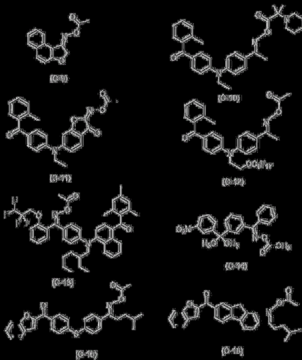
[化學式 9]
