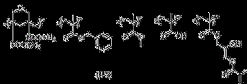
[化學式 17]
