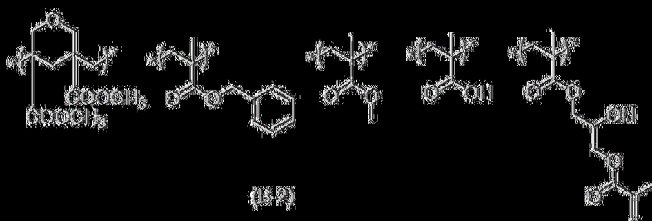
[化學式 17]
