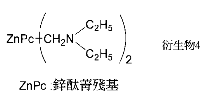
[化學式 13]
