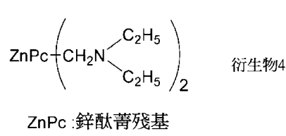
[化學式 13]
