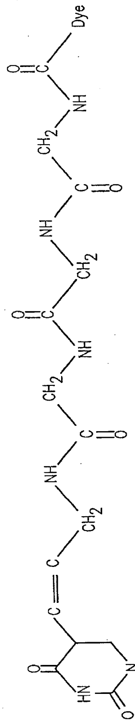
Tetraglycyl linker
