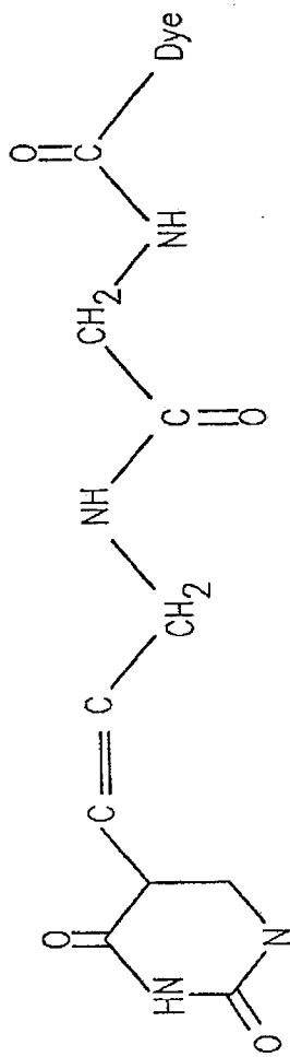
Diglycyl linker
