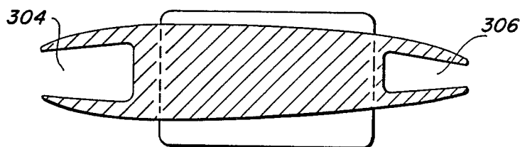
SECT S-S
