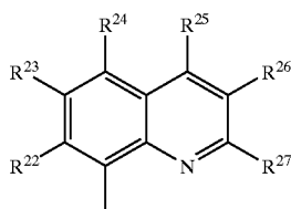
8-Quinolyl
