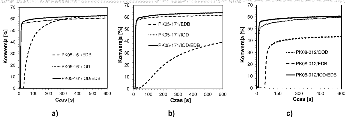
Wykres 50. Profile kinetyczne przedstawiające przebieg fotopolimeryzacji rodnikowej monomeru akrylanowego TMPTA dla dwu- i trójskładnikowych systemów inicjujących złożonych z soli diarylojodoniowej (IOD), aminy (EDB) oraz pochodnych 2-(dietyloamino)-4,6-difenylo-benzono-1,3-karbonitrylu a) PK05-161, b) PK05-171, c) PK08-012 przy 405 nm.
