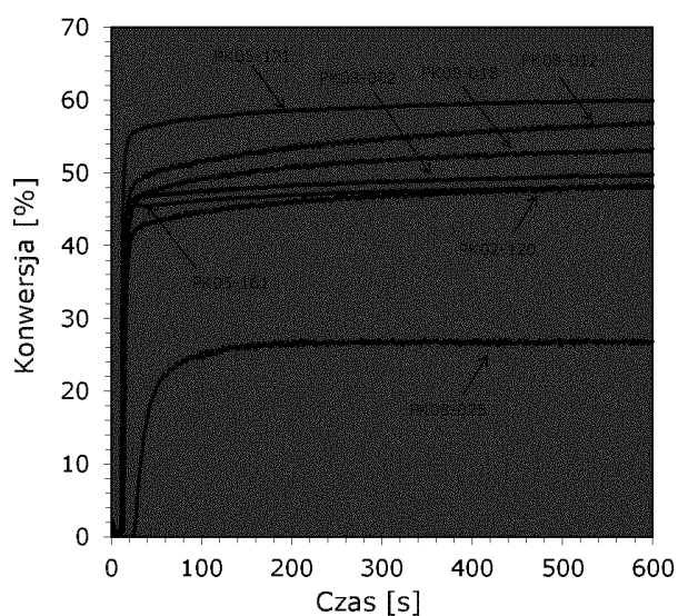
Wykres 36. Wybrane profile kinetyczne przedstawiające przebieg fotopolimeryzacji rodnikowej monomeru akrylanowego TMPTA dla systemu inicjującego złożonego z soli diarylojodoniowej + pochodne 2-(dietyloamino)-4,6-difenylo-benzeno-1,3-karbonitrylu (seria nr 3) przy 405 nm.
