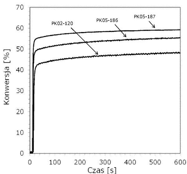
Wykres 37. Wybrane profile kinetyczne przedstawiające przebieg fotopolimeryzacji rodnikowej monomeru akrylanowego TMPTA dla systemu inicjującego złożonego z soli diarylojodoniowej + pochodne 2-(dietyloamino)-4,6-difenylo-benzeno-1,3-karbonitrylu (seria nr 4) przy 405 nm.
