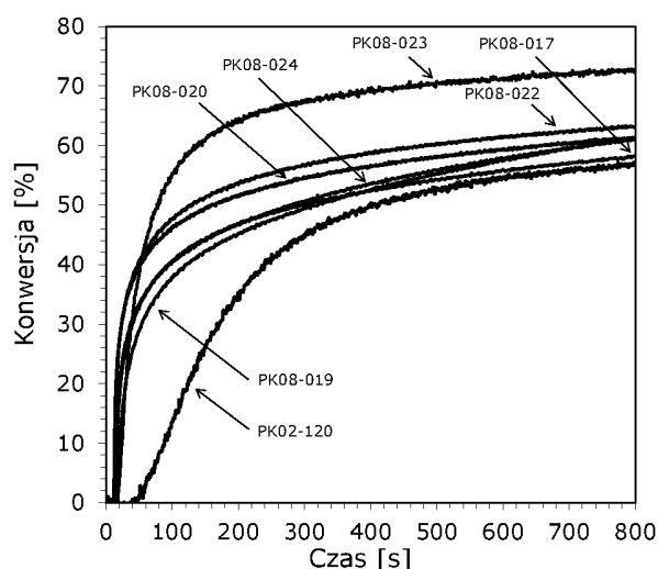
Wykres 25. Wybrane profile kinetyczne przedstawiające przebieg fotopolimeryzacji kationowej monomeru epoksydowego CADE dla systemu inicjującego sól diarylojodoniowa + pochodne 2-(dietyloamino)-4,6-difenylo-benzeno-1,3-karbonitrylu (seria nr 2) przy 420 nm.
