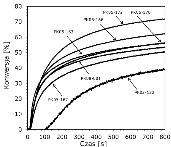
Wykres 28. Wybrane profile kinetyczne przedstawiające przebieg fotopolimeryzacji kationowej monomeru epoksydowego CADE dla systemu inicjującego sól diarylojodoniowa + pochodne 2-(dietyloamino)-4,6-difenylo-benzeno-1,3-karbonitrylu (seria nr 1) przy 455 nm.
