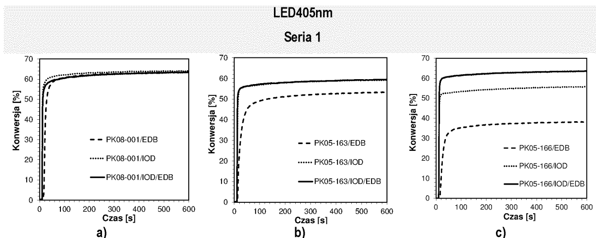
Wykres 46. Profile kinetyczne przedstawiające przebieg fotopolimeryzacji rodnikowej monomeru akrylanowego TMPTA dla dwu- i trójskładnikowych systemów inicjujących złożonych z soli diarylojodoniowej (IOD), aminy (EDB) oraz pochodnych 2-(dietyloamino)-4,6-difenylo-benzeno-1,3-karbonitrylu a) PK08-001, b) PK05-163, c) PK05-166 przy 405 nm.
