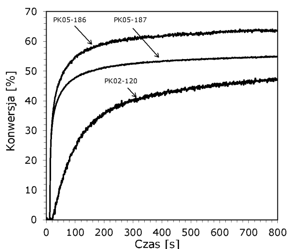
Wykres 23. Wybrane profile kinetyczne przedstawiające przebieg fotopolimeryzacji kationowej monomeru epoksydowego CADE dla systemu inicjującego sól diarylojodoniowa + pochodne 2-(dietyloamino)-4,6-difenylo-benzeno-1,3-karbonitrylu (seria nr 4) przy 405 nm.
