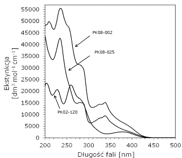
Wykres 5. Przykładowe widma absorpcji pochodnych 2-(dietyloamino)-4,6-difenylo-benzono-1,3-karbonitrylu w acetonitrylu – zestawienie porównawcze.
