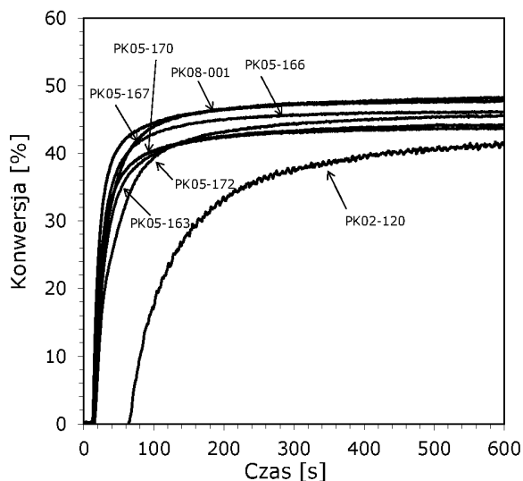
Wykres 42. Wybrane profile kinetyczne przedstawiające przebieg fotopolimeryzacji rodnikowej monomeru akrylanowego TMPTA dla systemu inicjującego złożonego z soli diarylojodoniowej + pochodne 2-(dietyloamino)-4,6-difenylo-benzeno-1,3-karbonitrylu (seria nr 1) przy 455 nm.
