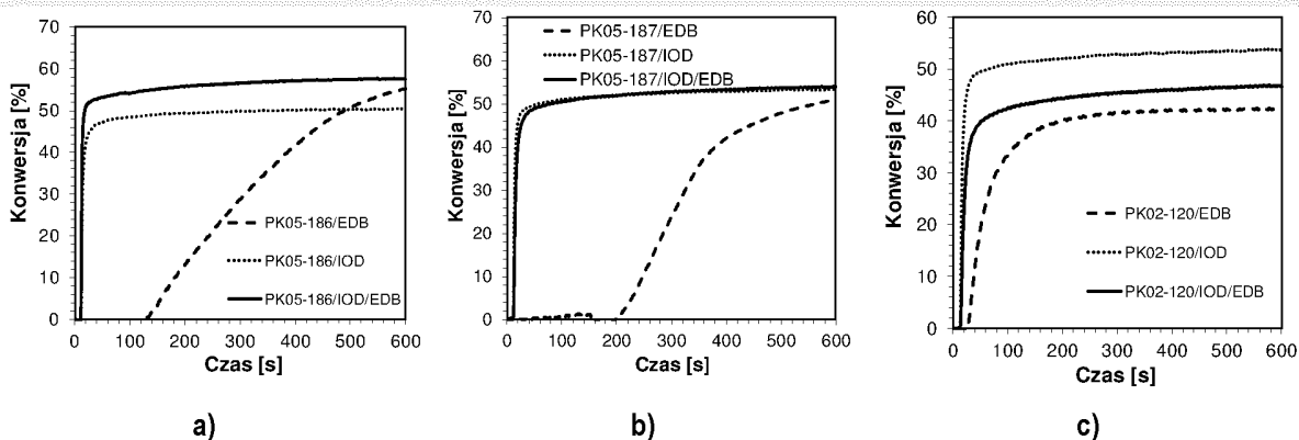
Wykres 59. Profile kinetyczne przedstawiające przebieg fotopolimeryzacji rodnikowej monomeru akrylanowego TMPTA dla dwu- i trójskładnikowych systemów inicjujących złożonych z soli diarylojodoniowej (IOD), aminy (EDB) oraz pochodnych 2-(dietyloamino)-4,6-difenylo-benzono-1,3-karbonitrylu a) PK05-186, b) PK05-187, c) PK02-120 przy 420 nm.
