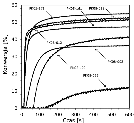
Wykres 44. Wybrane profile kinetyczne przedstawiające przebieg fotopolimeryzacji rodnicowej monomeru akrylanowego TMPTA dla systemu inicjującego złożonego z soli diarylojodoniowej + pochodne 2-(dietyloamino)-4,6-difenylo-benzeno-1,3-karbonitrylu (seria nr 3) przy 455 nm.
