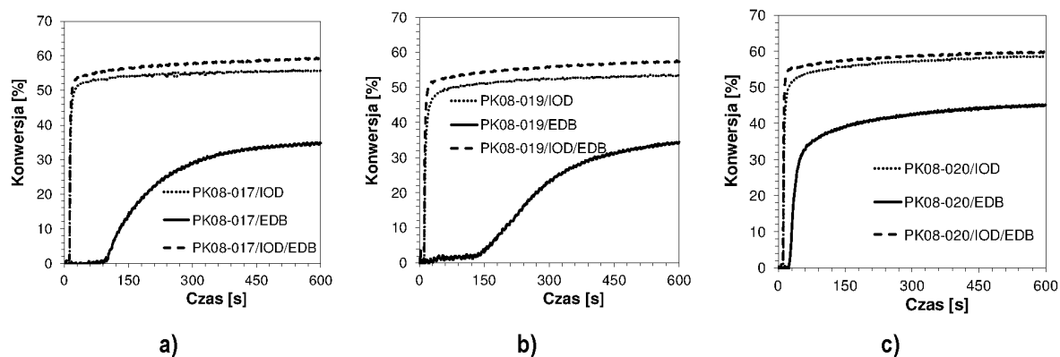
Wykres 60. Profile kinetyczne przedstawiające przebieg fotopolimeryzacji rodnikowej monomeru akrylanowego TMPTA dla dwu- i trójskładnikowych systemów inicjujących złożonych z soli diarylojodoniowej (IOD), aminy (EDB) oraz pochodnych 2-(dietyloamino)-4,6-difenylo-benzeno-1,3-karbonitrylu a) PK08-017, b) PK08-019, c) PK08-020 przy 455 nm.
