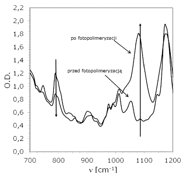
Wykres 19. Zmiany widma FT-IR dla kompozycji na bazie monomeru epoksydowego CADE przed i po procesie fotopolimeryzacji kationowej przy naświetlaniu diodą UV-LED 405 nm, przy użyciu inicjatora złożonego z soli diarylojodoniowej (1% wag.) + PK05-171 (0,1% wag.) (seria 3).
