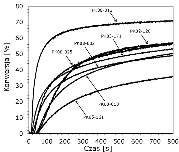
Wykres 26. Wybrane profile kinetyczne przedstawiające przebieg fotopolimeryzacji kationowej monomeru epoksydowego CADE dla systemu inicjującego sól diarylojodoniowa + pochodne 2-(dietyloamino)-4,6-difenylo-benzeno-1,3-karbonitrylu (seria nr 3) przy 420nm.
