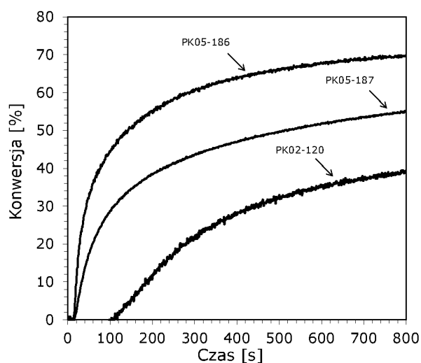
Wykres 31. Wybrane profile kinetyczne przedstawiające przebieg fotopolimeryzacji kationowej monomeru epoksydowego CADE dla systemu inicjującego sól diarylojodoniowa + pochodne 2-(dietyloamino)-4,6-difenylo-benzeno-1,3-karbonitrylu (seria nr 4) przy 455 nm.
