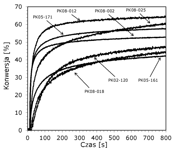
Wykres 22. Wybrane profile kinetyczne przedstawiające przebieg fotopolimeryzacji kationowej monomeru epoksydowego CADE dla systemu inicjującego sól diarylojodoniowa + pochodne 2-(dietyloamino)-4,6-difenylo-benzeno-1,3-karbonitrylu (seria nr 3) przy 405nm.
