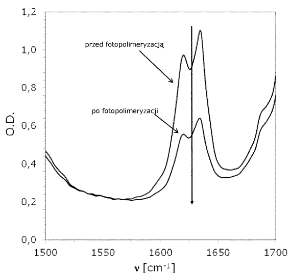
Wykres 32. Zmiana widma FT-IR dla kompozycji na bazie monomeru akrylanowego TMPTA przed i po procesie fotopolimeryzacji rodnikowej przy naświetlaniu diodą UV-LED 405 nm, przy użyciu inicjatora systemu inicjującego złożonego z soli diarylojodoniowej (1%wag.) + PK08-022 171 (0,1%wag.) (seria 2).
