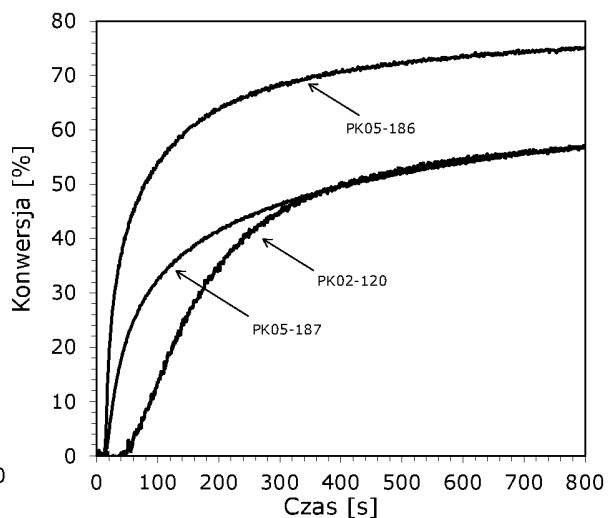
Wykres 27. Wybrane profile kinetyczne przedstawiające przebieg fotopolimeryzacji kationowej monomeru epoksydowego CADE dla systemu inicjującego sól diarylojodoniowa + pochodne 2-(dietyloamino)-4,6-difenylo-benzeno-1,3-karbonitrylu (seria nr 4) przy 420 nm.
