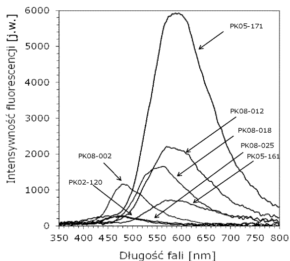
Wykres 13. Przykładowe widma fluorescencji pochodnych 2-(dietyloamino)-4,6-difenylo-benzenu-1,3-karbonitrylu w acetonitrylu przy wzbudzeniu światłem o długości fali równej 320 nm, przy czasie integracji 3000 ms (seria 3).
