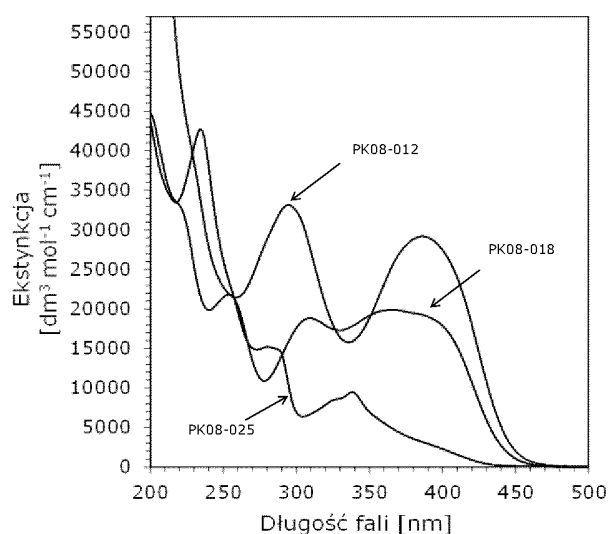
Wykres 6. Przykładowe widma absorpcji pochodnych 2-(dietyloamino)-4,6-difenylo-benzono-1,3-karbonitrylu w acetonitrylu – zestawienie porównawcze.
