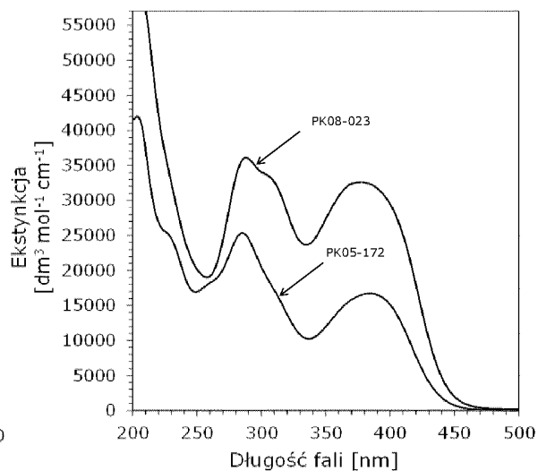
Wykres 8 Przykładowe widma absorpcji pochodnych 2-(dietyloamino)-4,6-difenylo-benzono-1,3-karbonitrylu w acetonitrylu – zestawienie porównawcze.
