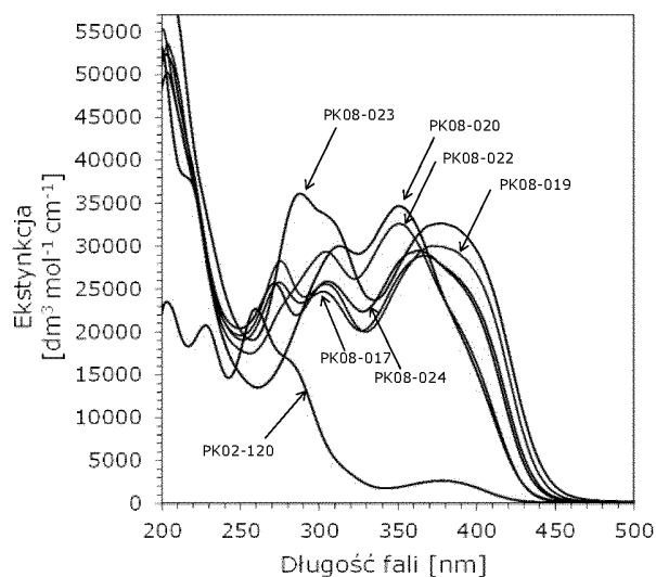
Wykres 2. Przykładowe widma absorpcji pochodnych 2-(dietyloamino)-4,6-difenylo-benzono-1,3-karbonitrylu w acetonitrylu (Seria 2).
