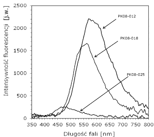
Wykres 15. Przykładowe widma fluorescencji pochodnych 2-(dietyloamino)-4,6-difenylo-benzono-1,3-karbonitrylu w acetonitrylu przy wzbudzeniu światłem o długości fali równej 320 nm, przy czasie integracji 3000 ms – zestawienie porównawcze.
