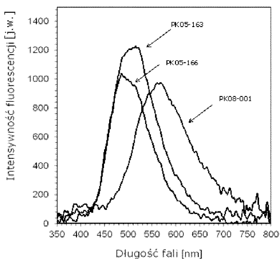
Wykres 11. Przykładowe widma fluorescencji pochodnych 2-(dietyloamino)-4,6-difenylo-benzono-1,3-karbonitrylu w acetonitrylu przy wzbudzeniu światłem o długości fali równej 320 nm, przy czasie integracji 3000 ms (seria 1).
