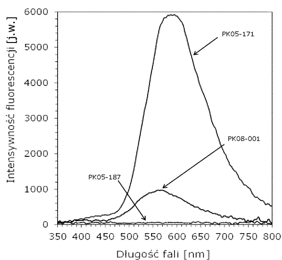
Wykres 14. Przykładowe widma fluorescencji pochodnych 2-(dietyloamino)-4,6-difenylo-benzono-1,3-karbonitrylu w acetonitrylu przy wzbudzeniu światłem o długości fali równej 320 nm, przy czasie integracji 3000 ms – zestawienie porównawcze.
