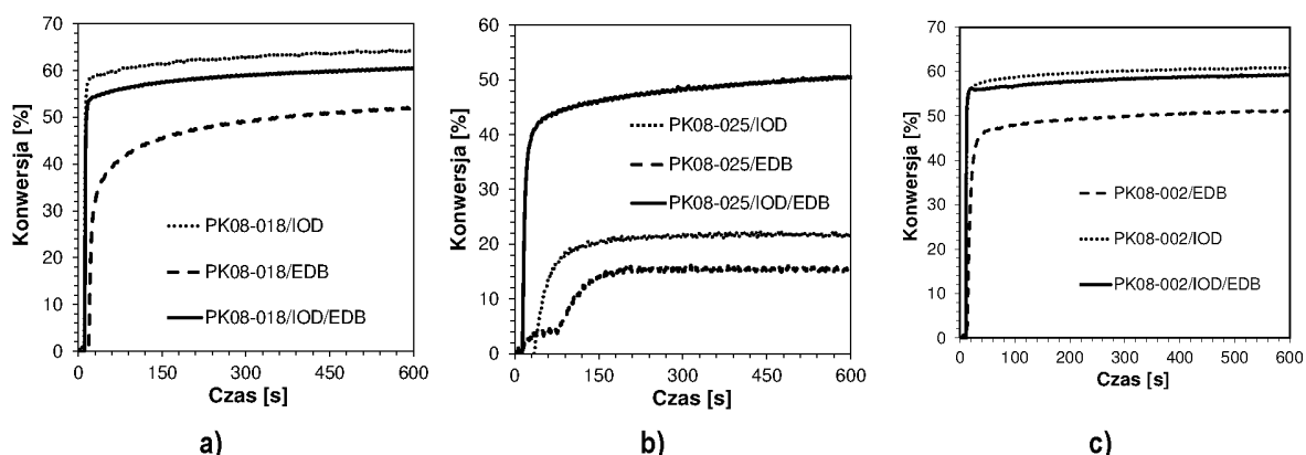
Wykres 51. Profile kinetyczne przedstawiające przebieg fotopolimeryzacji rodnikowej monomeru akrylanowego TMPTA dla dwu- i trójskładnikowych systemów inicjujących złożonych z soli diarylojodoniowej (IOD), aminy (EDB) oraz pochodnych 2-(dietyloamino)-4,6-difenyl-benzenu-1,3-karbonitrylu a) PK08-018, b) PK08-025, c) PK08-002 przy 405 nm.
