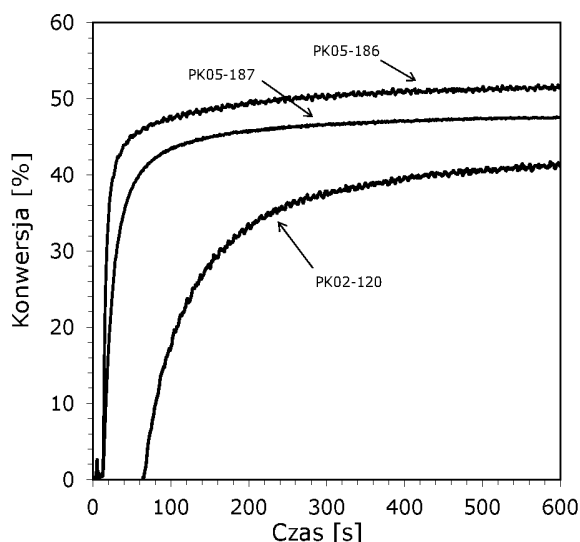
Wykres 45. Wybrane profile kinetyczne przedstawiające przebieg fotopolimeryzacji rodnicowej monomeru akrylanowego TMPTA dla systemu inicjującego złożonego z soli diarylojodoniowej + pochodne 2-(dietyloamino)-4,6-difenylo-benzeno-1,3-karbonitrylu (seria nr 4) przy 455 nm.
