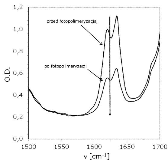
Wykres 33. Zmiana widma FT-IR dla kompozycji na bazie monomeru akrylanowego TMPTA przed i po procesie fotopolimeryzacji kationowej przy naświetlaniu diodą UV-LED 405 nm, przy użyciu inicjatora systemu inicjującego złożonego z soli diarylojodoniowej (1%wag.) + PK05-171 (0,1%wag.) (seria 3).
