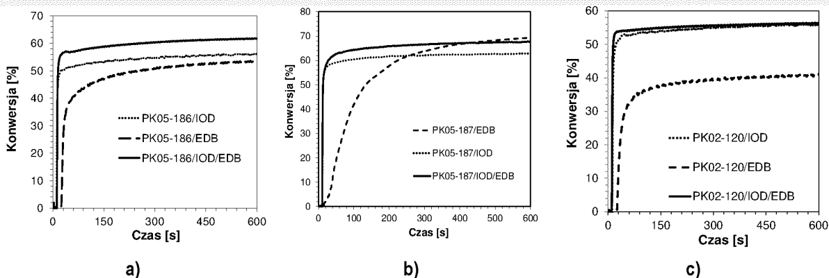
Wykres 52. Profile kinetyczne przedstawiające przebieg fotopolimeryzacji rodnikowej monomeru akrylanowego TMPTA dla dwu- i trójskładnikowych systemów inicjujących złożonych z soli diarylojodoniowej (IOD), aminy (EDB) oraz pochodnych 2-(dietyloamino)-4,6-difenyl-benzenu-1,3-karbonitrylu a) PK05-186, b) PK05-187, c) PK02-120 przy 405 nm.
