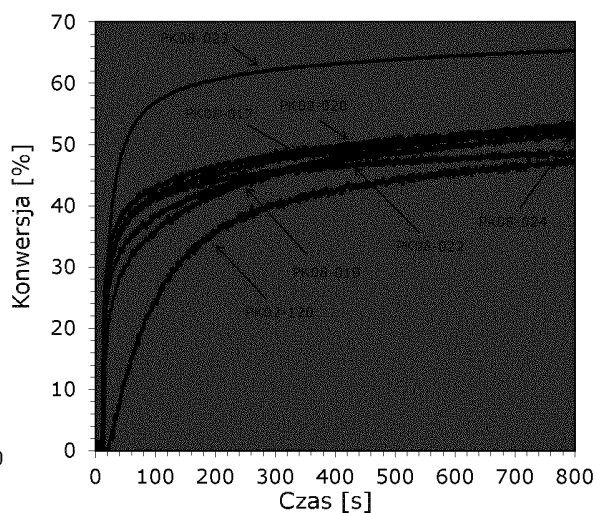
Wykres 21. Wybrane profile kinetyczne przedstawiające przebieg fotopolimeryzacji kationowej monomeru epoksydowego CADE dla systemu inicjującego sól diarylojodoniowa + pochodne 2-(dietyloamino)-4,6-difenylo-benzeno-1,3-karbonitrylu (seria nr 2) przy 405 nm.
