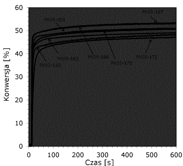
Wykres 34. Wybrane profile kinetyczne przedstawiające przebieg fotopolimeryzacji rodnikowej monomeru akrylanowego TMPTA dla systemu inicjującego złożonego z soli diarylojodoniowej + pochodne 2-(dietyloamino)-4,6-difenylo-benzeno-1,3-karbonitrylu (seria nr 1) przy 405 nm.
