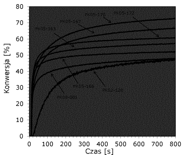
Wykres 20. Wybrane profile kinetyczne przedstawiające przebieg fotopolimeryzacji kationowej monomeru epoksydowego CADE dla systemu inicjującego sól diarylojodoniowa + pochodne 2-(dietyloamino)-4,6-difenylo-benzeno-1,3-karbonitrylu (seria nr 1) przy 405 nm.
