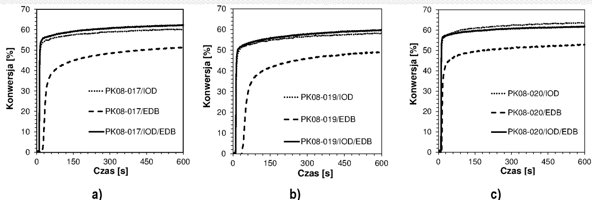
Wykres 48. Profile kinetyczne przedstawiające przebieg fotopolimeryzacji rodnikowej monomeru akrylanowego TMPTA dla dwu- i trójskładnikowych systemów inicjujących złożonych z soli diarylojodoniowej (IOD), aminy (EDB) oraz pochodnych 2-(dietyloamino)-4,6-difenylo-benzono-1,3-karbonitrylu a) PK08-017, b) PK08-019, c) PK08-020 przy 405 nm.
