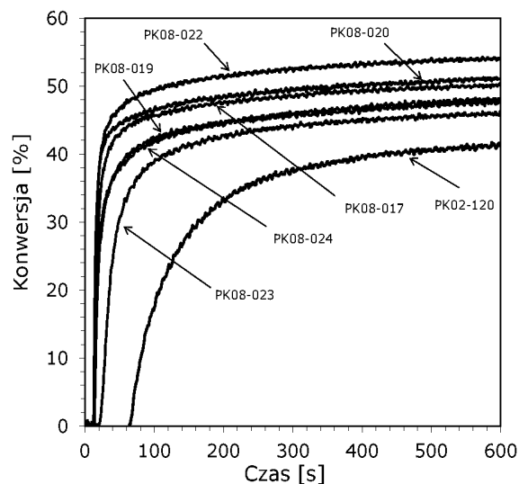
Wykres 43. Wybrane profile kinetyczne przedstawiające przebieg fotopolimeryzacji rodnikowej monomeru akrylanowego TMPTA dla systemu inicjującego złożonego z soli diarylojodoniowej + pochodne 2-(dietyloamino)-4,6-difenylo-benzeno-1,3-karbonitrylu (seria nr 2) przy 455 nm.
