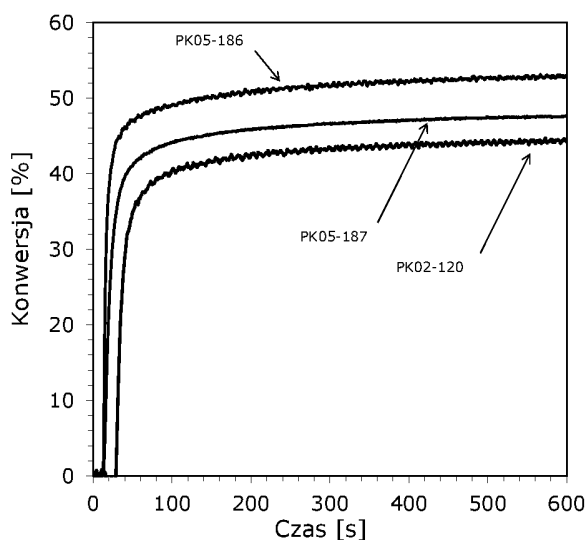
Wykres 41. Wybrane profile kinetyczne przedstawiające przebieg fotopolimeryzacji rodnikowej monomeru akrylanowego TMPTA dla systemu inicjującego złożonego z soli diarylojodoniowej + pochodne 2-(dietyloamino)-4,6-difenylo-benzeno-1,3-karbonitrylu (seria nr 4) przy 420 nm.
