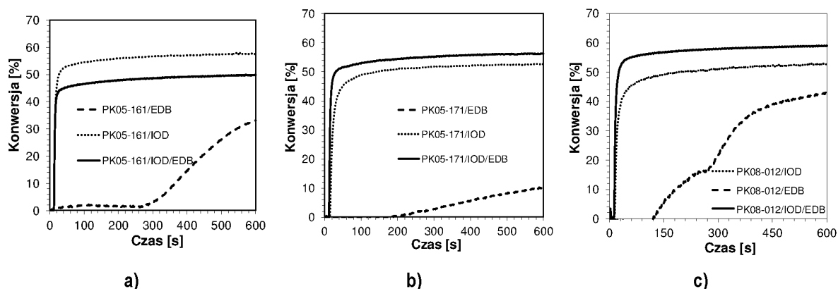
Wykres 57. Profile kinetyczne przedstawiające przebieg fotopolimeryzacji rodnikowej monomeru akrylanowego TMPTA dla dwu- i trójskładnikowych systemów inicjujących złożonych z soli diarylojodoniowej (IOD), aminy (EDB) oraz pochodnych 2-(dietyloamino)-4,6-difenylo-benzono-1,3-karbonitrylu a) PK05-161, b) PK05-171, c) PK08-012 przy 420 nm.
