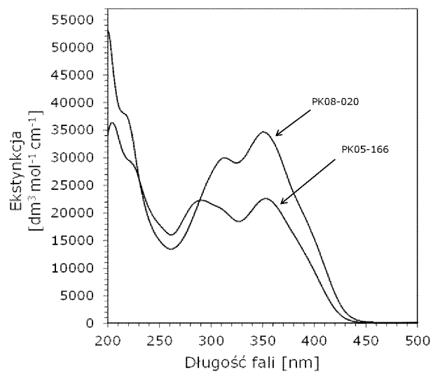
Wykres 7. Przykładowe widma absorpcji pochodnych 2-(dietyloamino)-4,6-difenylo-benzono-1,3-karbonitrylu w acetonitrylu – zestawienie porównawcze.
