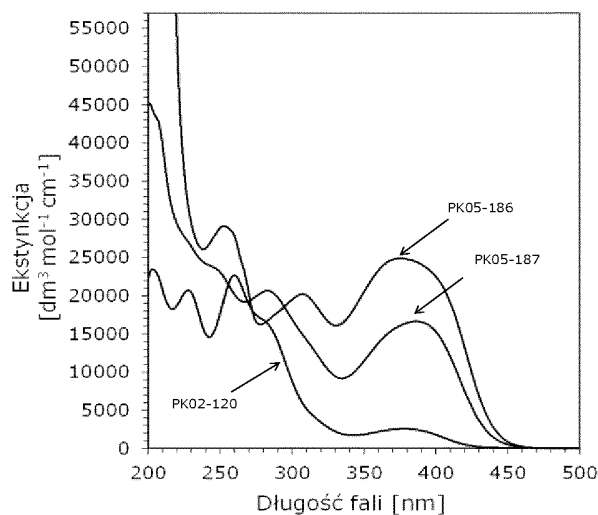
Wykres 4. Przykładowe widma absorpcji pochodnych 2-(dietyloamino)-4,6-difenylo-benzono-1,3-karbonitrylu w acetonitrylu (seria 4).
