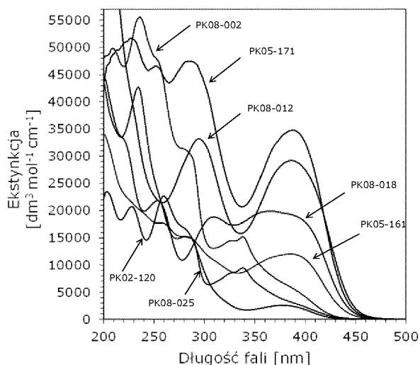
Wykres 3. Przykładowe widma absorpcji pochodnych 2-(dietyloamino)-4,6-difenylo-benzono-1,3-karbonitrylu w acetonitrylu (seria 3).
