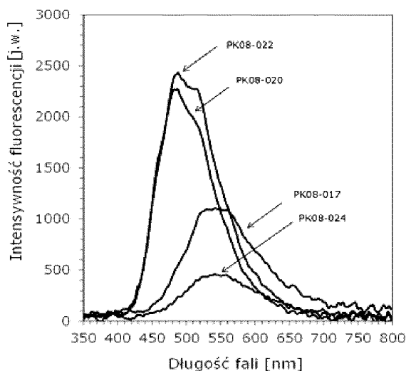
Wykres 12. Przykładowe widma fluorescencji pochodnych 2-(dietyloamino)-4,6-difenylo-benzono-1,3-karbonitrylu w acetonitrylu przy wzbudzeniu światłem o długości fali równej 320 nm, przy czasie integracji 3000 ms (seria 2).
