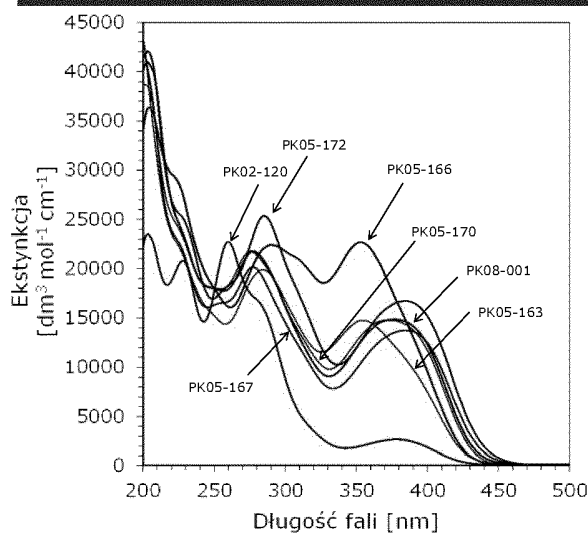
Wykres 1. Przykładowe widma absorpcji pochodnych 2-(dietyloamino)-4,6-difenylo-benzono-1,3-karbonitrylu w acetonitrylu (seria 1).
