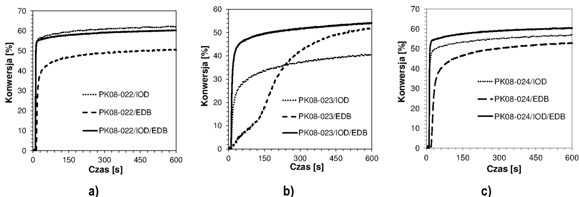
Wykres 49. Profile kinetyczne przedstawiające przebieg fotopolimeryzacji rodnikowej monomeru akrylanowego TMPTA dla dwu- i trójskładnikowych systemów inicjujących złożonych z soli diarylojodoniowej (IOD), aminy (EDB) oraz pochodnych 2-(dietyloamino)-4,6-difenylo-benzono-1,3-karbonitrylu a) PK08-022, b) PK08-023, c) PK08-024 przy 405 nm.
