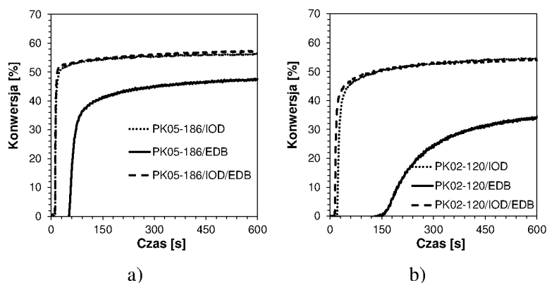
Wykres 63. Profile kinetyczne przedstawiające przebieg fotopolimeryzacji rodnikowej monomeru akrylanowego TMPTA dla dwu- i trójskładnikowych systemów inicjujących złożonych z soli diarylojodoniowej (IOD), aminy (EDB) oraz pochodnych 2-(dietyloamino)-4,6-difenylo-benzeno-1,3-karbonitrylu a) PK05-186, b) PK02-120 przy 455 nm.
