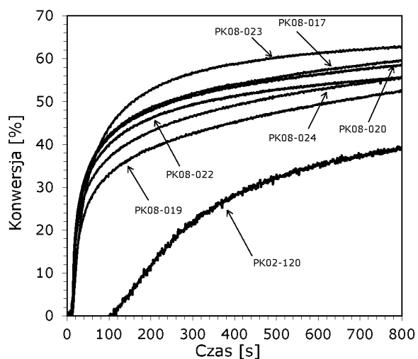
Wykres 29. Wybrane profile kinetyczne przedstawiające przebieg fotopolimeryzacji kationowej monomeru epoksydowego CADE dla systemu inicjującego sól diarylojodoniowa + pochodne 2-(dietyloamino)-4,6-difenylo-benzeno-1,3-karbonitrylu (seria nr 2) przy 455 nm.
