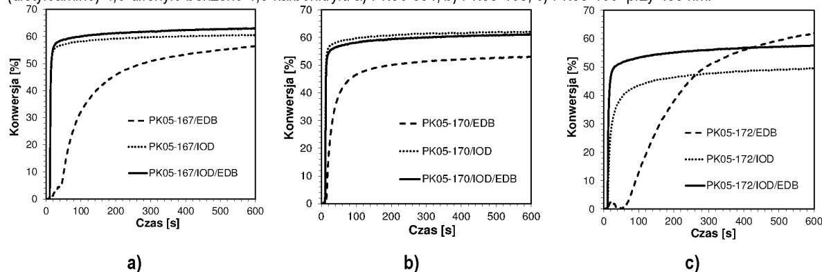
Wykres 47. Profile kinetyczne przedstawiające przebieg fotopolimeryzacji rodnikowej monomeru akrylanowego TMPTA dla dwu- i trójskładnikowych systemów inicjujących złożonych z soli diarylojodoniowej (IOD), aminy (EDB) oraz pochodnych 2-(dietyloamino)-4,6-difenylo-benzeno-1,3-karbonitrylu a) PK05-167, b) PK05-170, c) PK05-172 przy 405 nm.
