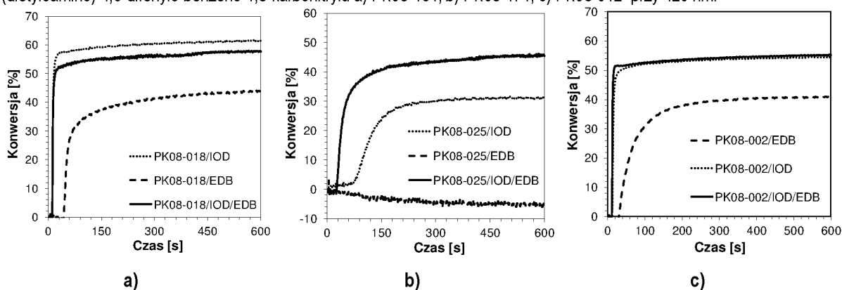
Wykres 58. Profile kinetyczne przedstawiające przebieg fotopolimeryzacji rodnikowej monomeru akrylanowego TMPTA dla dwu- i trójskładnikowych systemów inicjujących złożonych z soli diarylojodoniowej (IOD), aminy (EDB) oraz pochodnych 2-(dietyloamino)-4,6-difenylo-benzono-1,3-karbonitrylu a) PK08-018, b) PK08-025, c) PK08-002 przy 420 nm.
