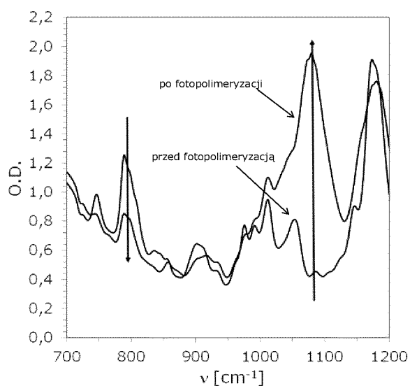
Wykres 18. Zmiany widma FT-IR dla kompozycji na bazie monomeru epoksydowego CADE przed i po procesie fotopolimeryzacji kationowej przy naświetlaniu diodą UV-LED 405 nm, przy użyciu inicjatora systemu inicjującego inicjatora złożonego z soli diarylojodoniowej (1% wag.) + PK08-012 (0,1% wag.) (seria 3).
