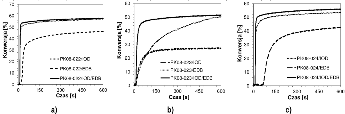
Wykres 56. Profile kinetyczne przedstawiające przebieg fotopolimeryzacji rodnikowej monomeru akrylanowego TMPTA dla dwu- i trójskładnikowych systemów inicjujących złożonych z soli diarylojodoniowej (IOD), aminy (EDB) oraz pochodnych 2-(dietyloamino)-4,6-difenylo-benzono-1,3-karbonitrylu a) PK08-022, b) PK08-023, c) PK08-024 przy 420 nm.
