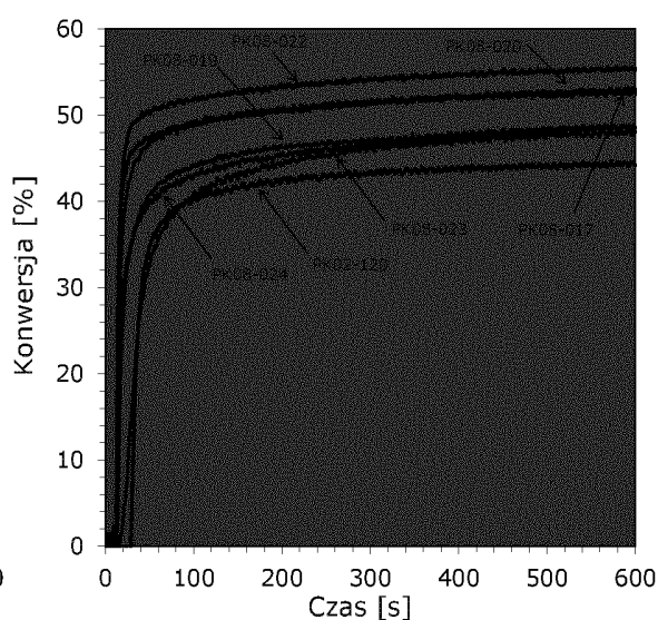
Wykres 39. Wybrane profile kinetyczne przedstawiające przebieg fotopolimeryzacji rodnikowej monomeru akrylanowego TMPTA dla systemu inicjującego złożonego z soli diarylojodoniowej + pochodne 2-(dietyloamino)-4,6-difenylo-benzeno-1,3-karbonitrylu (seria nr 2) przy 420 nm.
