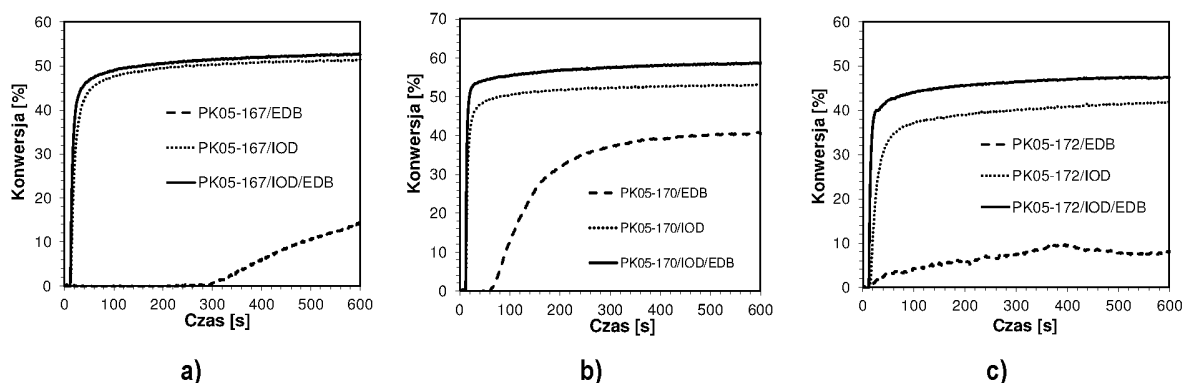
Wykres 54. Profile kinetyczne przedstawiające przebieg fotopolimeryzacji rodnikowej monomeru akrylanowego TMPTA dla dwu- i trójskładnikowych systemów inicjujących złożonych z soli diarylojodoniowej (IOD), aminy (EDB) oraz pochodnych 2-(dietyloamino)-4,6-difenylo-benzono-1,3-karbonitrylu a) PK05-167, b) PK05-170, c) PK05-172 przy 420 nm.
