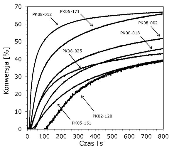
Wykres 30. Wybrane profile kinetyczne przedstawiające przebieg fotopolimeryzacji kationowej monomeru epoksydowego CADE dla systemu inicjującego sól diarylojodoniowa + pochodne 2-(dietyloamino)-4,6-difenylo-benzeno-1,3-karbonitrylu (seria nr 3) przy 455 nm.
