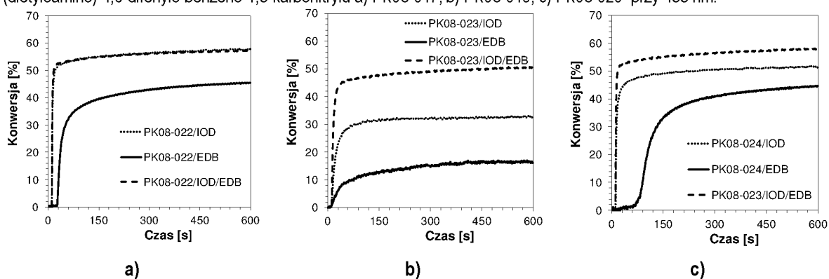
Wykres 61. Profile kinetyczne przedstawiające przebieg fotopolimeryzacji rodnikowej monomeru akrylanowego TMPTA dla dwu- i trójskładnikowych systemów inicjujących złożonych z soli diarylojodoniowej (IOD), aminy (EDB) oraz pochodnych 2-(dietyloamino)-4,6-difenylo-benzeno-1,3-karbonitrylu a) PK08-022, b) PK08-023, c) PK08-024 przy 455 nm.
