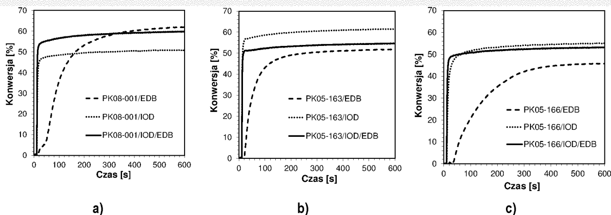
Wykres 53. Profile kinetyczne przedstawiające przebieg fotopolimeryzacji rodnikowej monomeru akrylanowego TMPTA dla dwu- i trójskładnikowych systemów inicjujących złożonych z soli diarylojodoniowej (IOD), aminy (EDB) oraz pochodnych 2-(dietyloamino)-4,6-difenyl-benzenu-1,3-karbonitrylu a) PK08-001, b) PK05-163, c) PK05-166 przy 420 nm.
