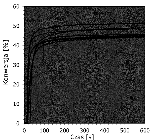
Wykres 38. Wybrane profile kinetyczne przedstawiające przebieg fotopolimeryzacji rodnikowej monomeru akrylanowego TMPTA dla systemu inicjującego złożonego z soli diarylojodoniowej + pochodne 2-(dietyloamino)-4,6-difenylo-benzeno-1,3-karbonitrylu (seria nr 1) przy 420 nm.
