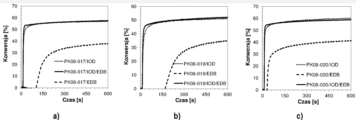
Wykres 55. Profile kinetyczne przedstawiające przebieg fotopolimeryzacji rodnikowej monomeru akrylanowego TMPTA dla dwu- i trójskładnikowych systemów inicjujących złożonych z soli diarylojodoniowej (IOD), aminy (EDB) oraz pochodnych 2-(dietyloamino)-4,6-difenylo-benzono-1,3-karbonitrylu a) PK08-017, b) PK08-019, c) PK08-020 przy 420 nm.
