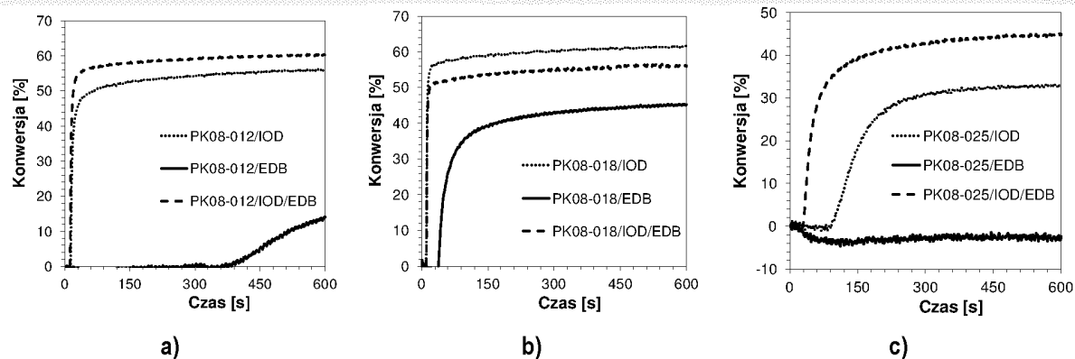
Wykres 62. Profile kinetyczne przedstawiające przebieg fotopolimeryzacji rodnikowej monomeru akrylanowego TMPTA dla dwu- i trójskładnikowych systemów inicjujących złożonych z soli diarylojodoniowej (IOD), aminy (EDB) oraz pochodnych 2-(dietyloamino)-4,6-difenylo-benzeno-1,3-karbonitrylu a) PK08-012, b) PK08-018, c) PK08-025 przy 455 nm.
