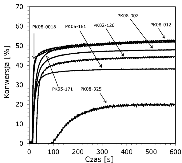
Wykres 40. Wybrane profile kinetyczne przedstawiające przebieg fotopolimeryzacji rodnikowej monomeru akrylanowego TMPTA dla systemu inicjującego złożonego z soli diarylojodoniowej + pochodne 2-(dietyloamino)-4,6-difenylo-benzeno-1,3-karbonitrylu (seria nr 3) przy 420 nm.
