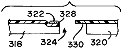
FIG. 37
