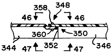
FIG. 45
