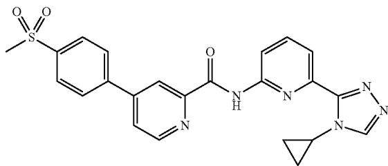
N-(6-(4-cyclopropyl-4H-1,2,4-triazol-3-yl)pyridin-2- yl)-4-(4-(methylsulfonyl)-phenyl)picolinamide
