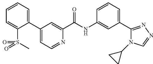
N-(3-(4-cyclopropyl-4H-1,2,4-triazol-3-yl)phenyl)-4-(2-(methylsulfonyl)phenyl)picolinamide
