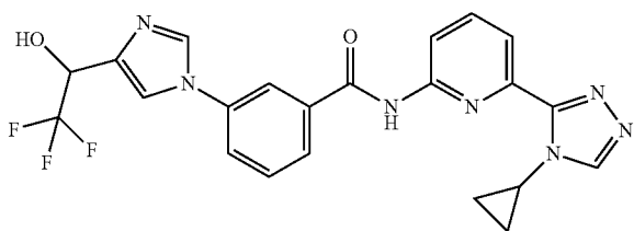
N-(6-(4-cyclopropyl-4H-1,2,4-triazol-3-yl)pyridin-2-yl)-3-(4-(2,2,2-trifluoro-1-hydroxyethyl)-1H-imidazol-1-yl)benzamide
