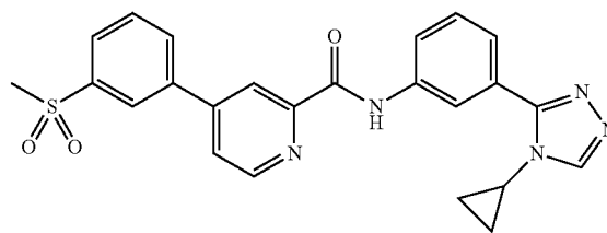
N-(3-(4-cyclopropyl-4H-1,2,4-triazol-3-yl)phenyl)-4-(3-(methylsulfonyl)phenyl)picolinamide
