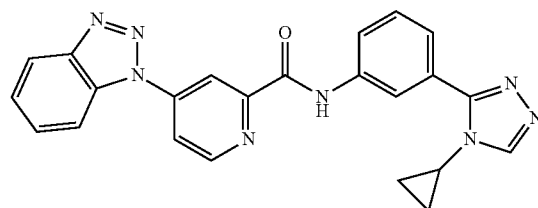
4-(1H-benzo[d][1,2,3]triazol-1-yl)-N-(3-(4-cyclopropyl-4H-1,2,4-triazol-3-yl)phenyl)picolinamide
