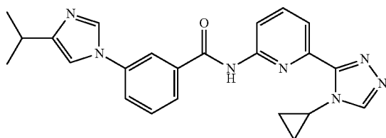
N-(6-(4-cyclopropyl-4H-1,2,4-triazol-3-yl)pyridin-2-yl)-3-(4-isopropyl-1H-imidazol-1-yl)benzamide
