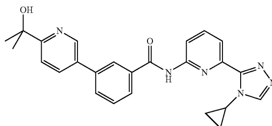
N-(6-(4-cyclopropyl-4H-1,2,4-triazol-3-yl)pyridin-2-yl)-3-(6-(2-hydroxypropan-2-yl)pyridin-3-yl)benzamide
