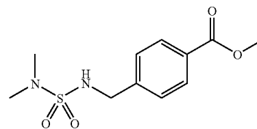
Methyl 4-(((dimethylamino)sulfonyl)amino)methyl)benzoate
