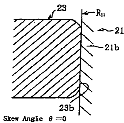
FIG. 5B(PRIOR ART)
