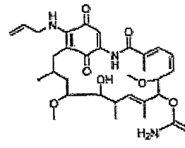
17-AAG
