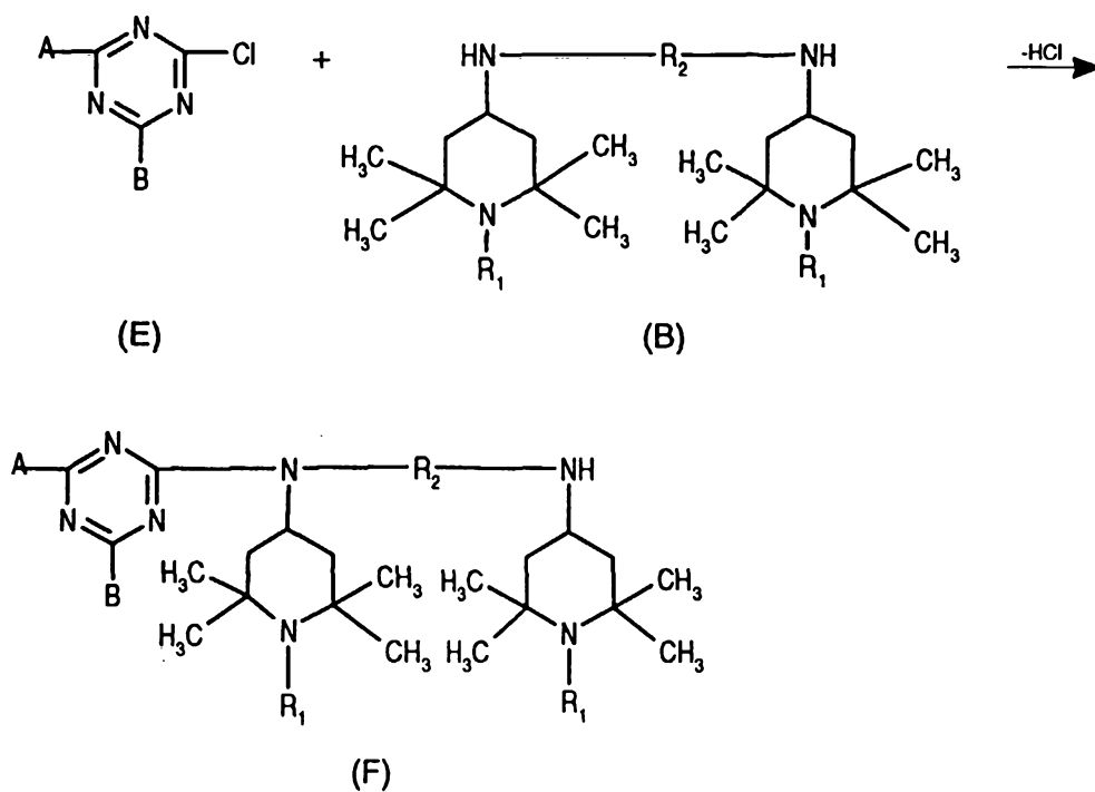
Scheme I-1:
