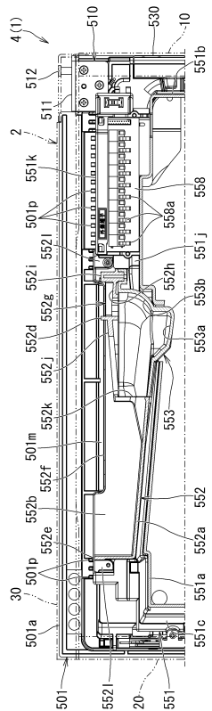
B-B断面図
