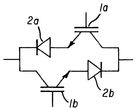
FIG. 25b (Prior Art)
